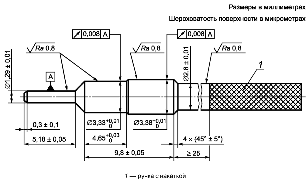
Рисунок 5 — Проходной калибр соединительного гнезда DF-1
