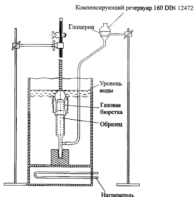
Рис. 5.4.6.6.1-1 Аппарат для определения содержания диффузионного водорода
