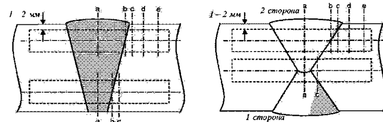
Рис. 6.4.4.3 Схема вырезки и расположения надреза на образцах для испытаний на ударный изгиб для технологических процессов сварки с погонной энергией > 50 \text{ кДж/см} :
