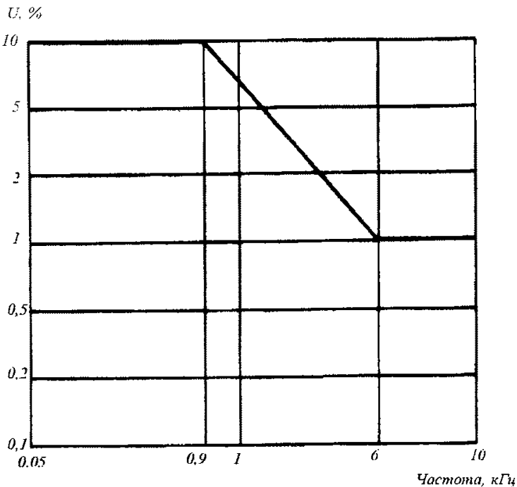
Рис. 6.2.1 Кривая испытательного напряжения при проверке оборудования на устойчивость к низкочастотным кондуктивным помехам
