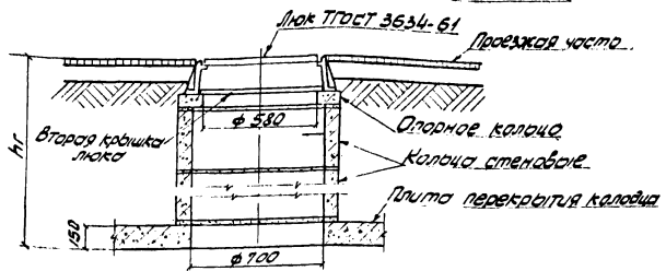
II Горловина колодца для временной нагрузки H-18
