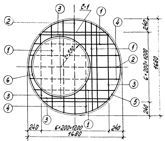
План нижней арматуры
