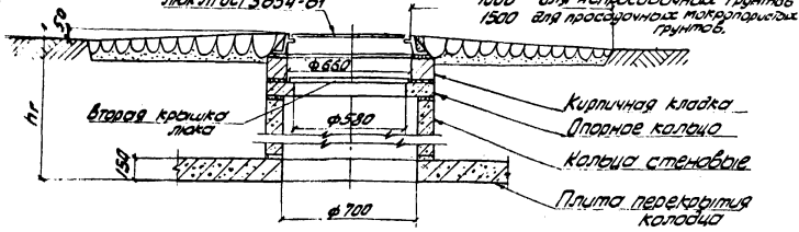
I Горловина колодца для временной нагрузки 500 кг/м²
