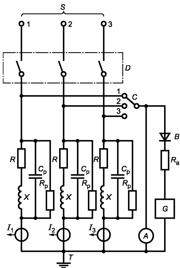
S — источник питания; X — катушки индуктивности; D — испытуемый контактор; B — диод; R_p — параллельные активные сопротивления; C — переключатель выбора фазы; C_p — параллельные конденсаторы; I_1, I_2, I_3 — датчики тока; A — регистрирующий прибор; R_a — резистор; G — высоковольтный генератор; R — активные сопротивления цепи нагрузки
