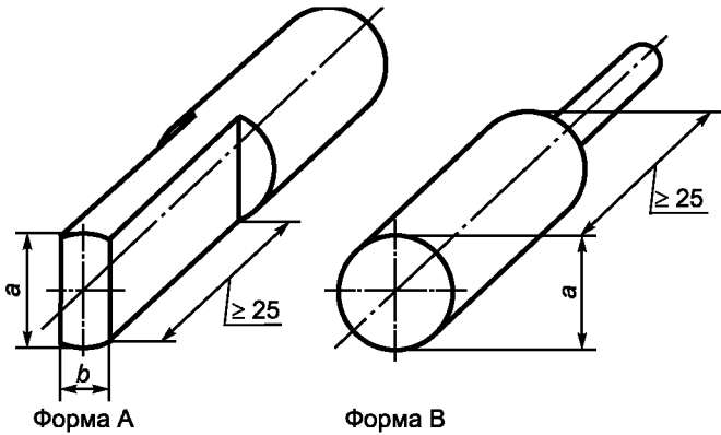
Рисунок 5 — Щупы (см. 9.2.4.5)
