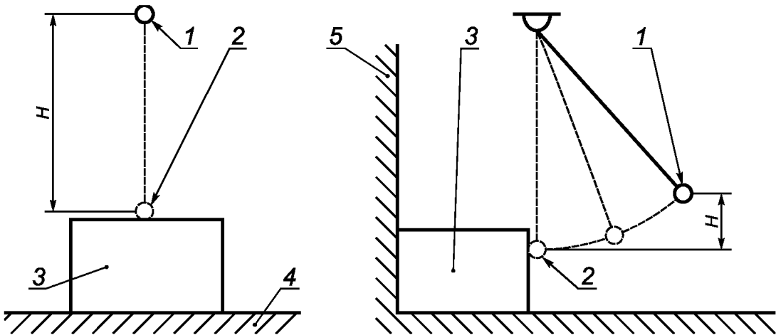
1 — начальное положение шарика; 2 — ударное положение шарика; 3 — испытуемый образец; 4 — жесткая опорная поверхность; 5 — жесткая задняя поверхность; H = 1300\text{ мм}
