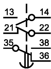
Три контактных элемента
