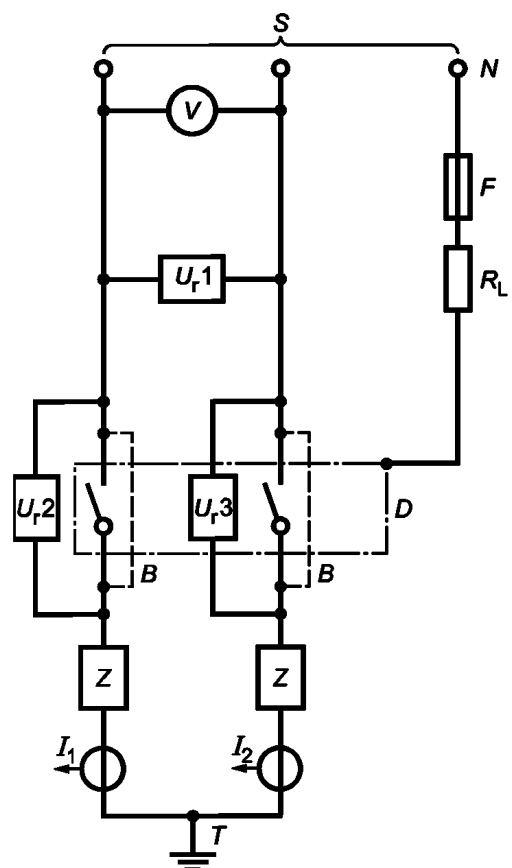
S — источник питания; U_{r1} , U_{r2} , U_{r3} — датчики напряжения; V — вольтметр; N — нейтраль (искусственная нейтраль); F — плавкий элемент; Z — цепь нагрузки; R_L — токоограничивающее сопротивление; D — испытуемый аппарат (с присоединенными проводниками); B — переключки для настройки контура; I_1 , I_2 — датчики тока; T — точка заземления (на стороне нагрузки или питания)
