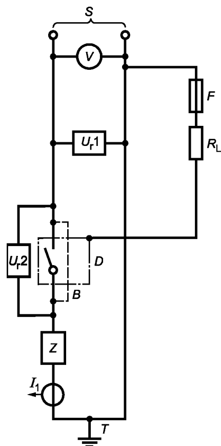
S — питание; U_{r1} , U_{r2} — датчики напряжения; F — плавкий элемент; Z — цепь нагрузки; R_L — токоограничивающее сопротивление; D — испытуемый аппарат (с присоединенными проводниками); B — переключки для настройки контура; I_1 — датчик тока; T — точка заземления (на стороне нагрузки или питания)
