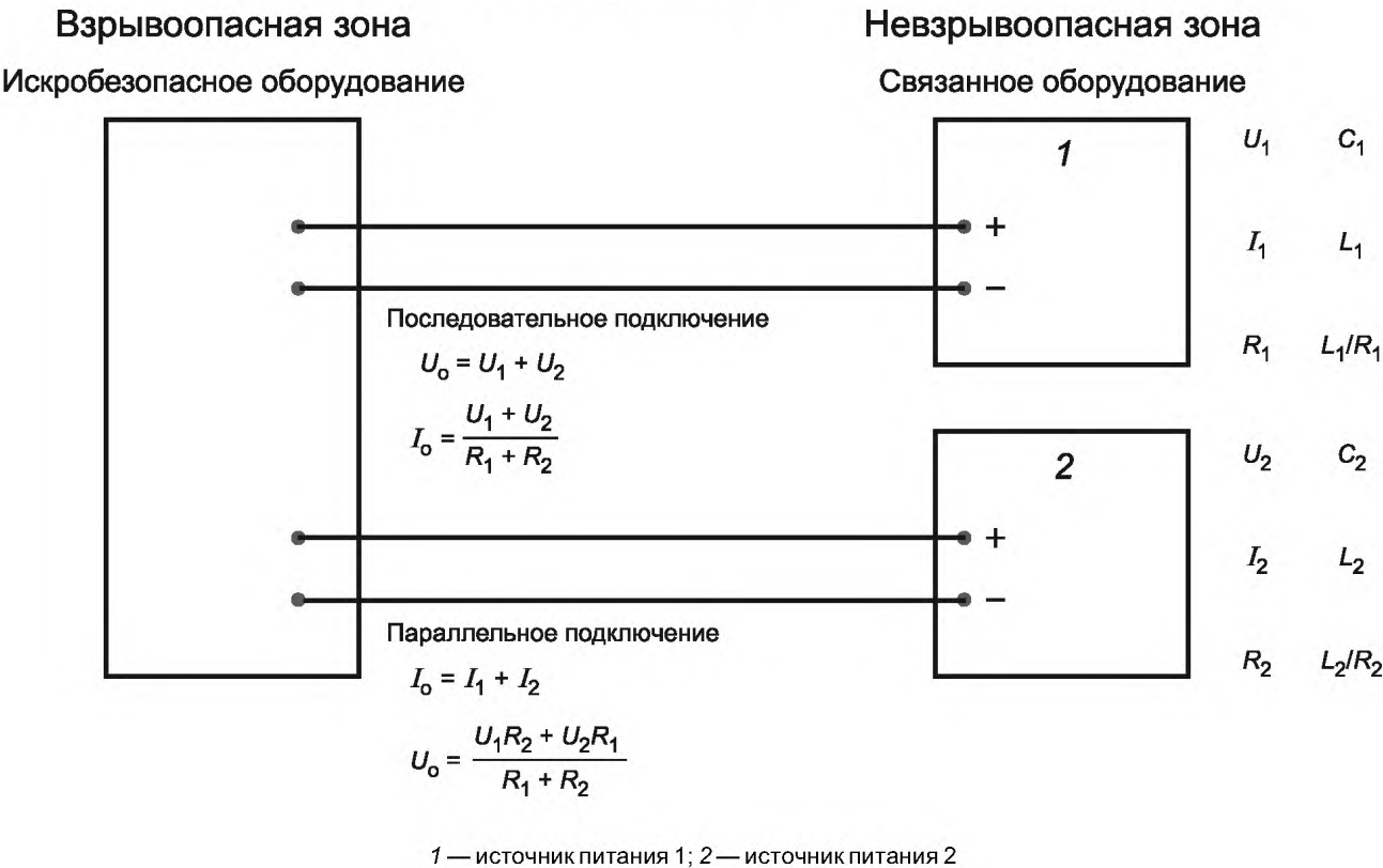
Рисунок D.3 — Источники питания, подключенные произвольно
