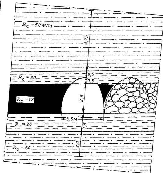
Рис. 26. Расчетная схема к примеру 4
