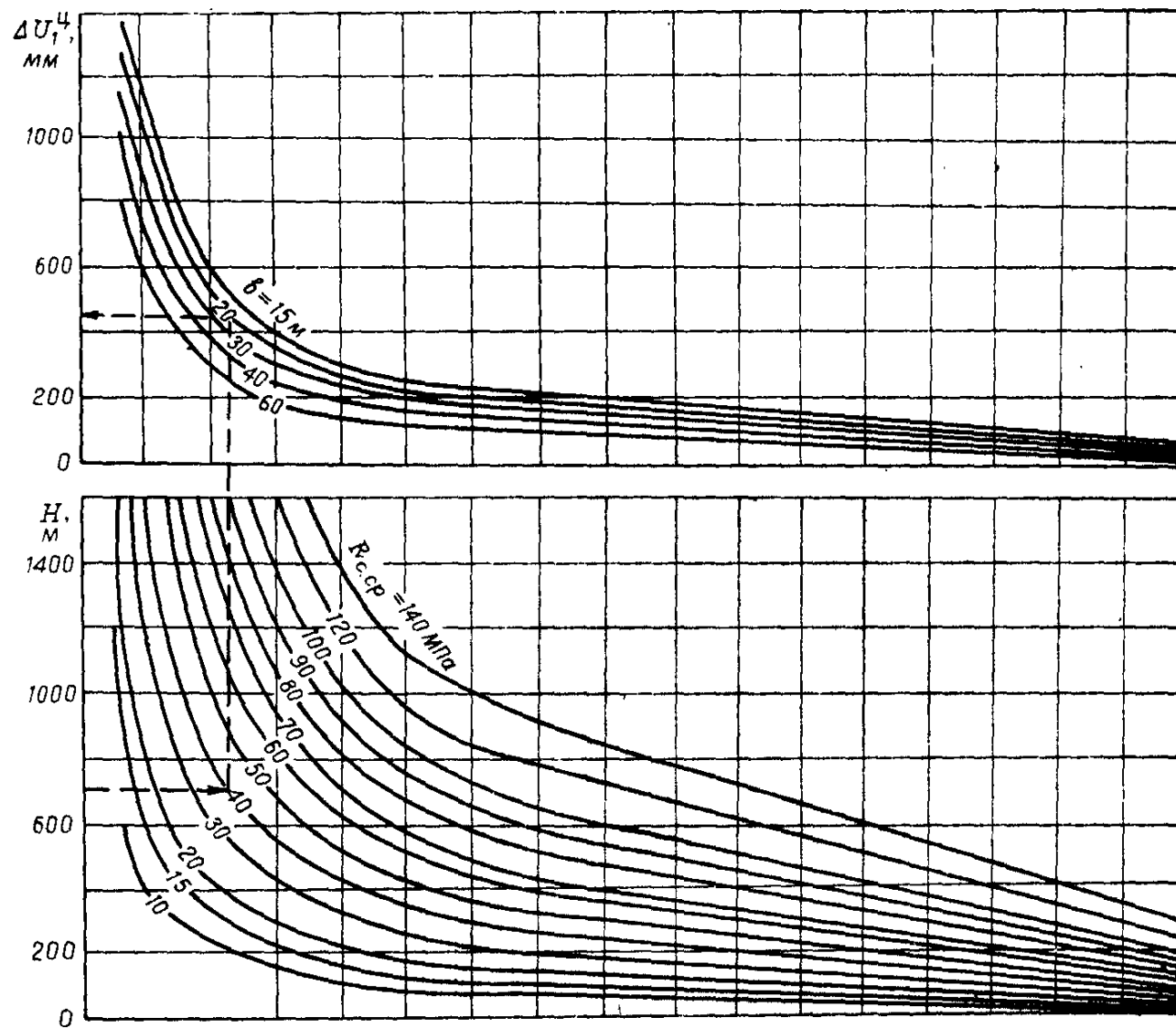
Рис. 10. Номограмма для определения \Delta U_1^4
