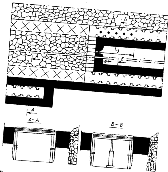
Рис. 25. Схема проведения выработок впрысчку к выработанному пространству
