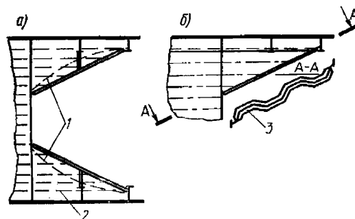
Рис. 2.5.1 Окончания продольных переборок:
