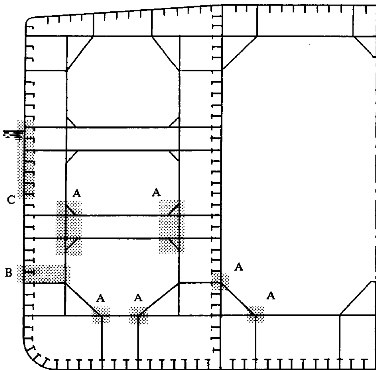
Рис. 2.2.1-7 Районы концентрации напряжений в элементах рамных шпангоутов танкеров: А — концентрация напряжений в местах окончания книц и аналогичных им конструкциях; В — концентрация напряжений в конструкциях, испытывающих напряжения среза; С — местная концентрация напряжений в связях между продольными ребрами жесткости и рамными шпангоутами
