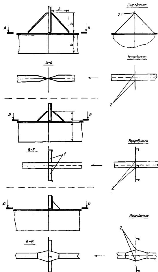
Рис. 2.2.1.4 Соединения вертикального килея и днищевых стрингеров с поперечными переборками, а также флоров с продольными переборками:
