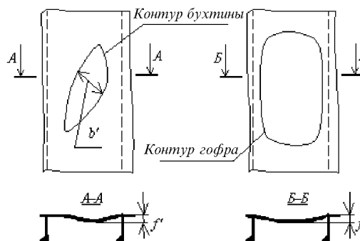
Рис. 3.3.3.1 Измерение параметров бухтины и гофра
