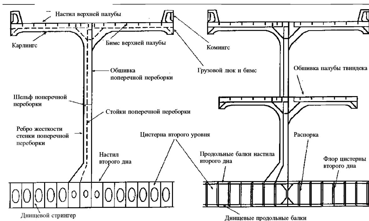
Рис. 2.2.1-4 Конструкция водонепроницаемой переборки сухогрузов
