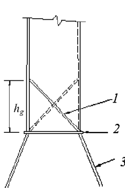
Рис. 1.4.2-1 Симметричные шедерные листы: 1 — шедерный лист; 2 — горизонтальный/наклонный лист опоры (полки) нижней опоры для переборки; 3 — вертикальная/наклонная опорная стенка нижней опоры для переборки
