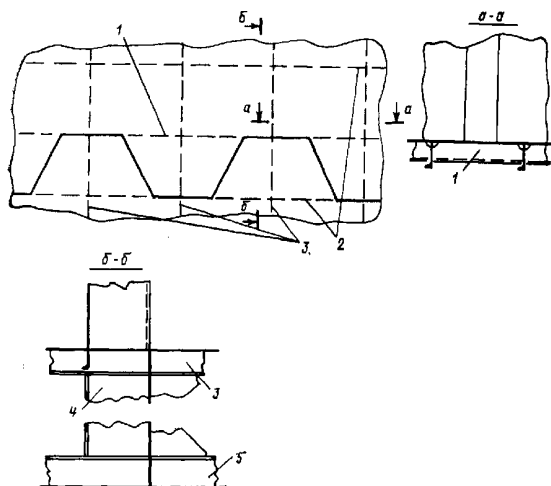
Рис. 2.5.9.1 Подкрепление настила второго дна под гофрированными переборками:
