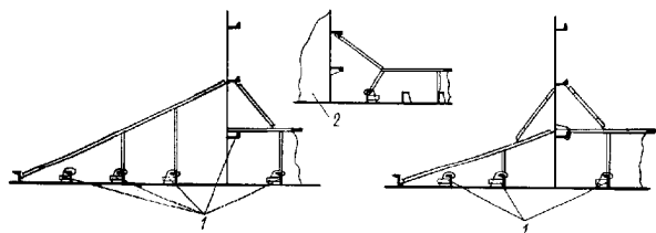
Рис. 2.3.5.5 Окончание бортовых стрингеров: 1 — заделки; 2 — платформа
