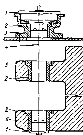
Рис. 5.2-2 Проверка соосности неподвижных составных частей рулевых устройств:
