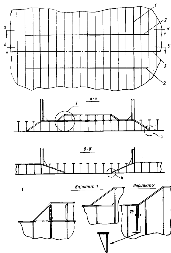
Рис. 2.2.1.5 Перевязка продольных балок машинного фундамента и вертикального килея:
