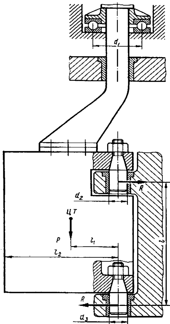
Рис. 6.4 Схема для расчета усилия поворота рулевого устройства
