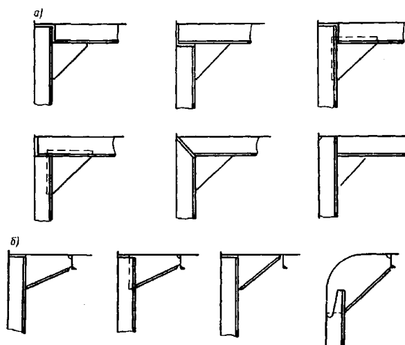
Рис. 2.3.2.1 Соединение концов шпангоутов с верхней палубой при поперечной ( а ) и продольной ( б ) системах набора палубы
