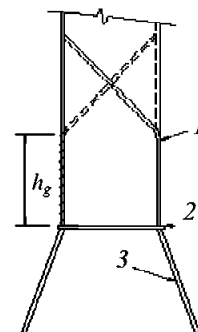
Рис. 1.4.2-3 Симметричные гассетный/шедерный листы: 1 — гассетный/шедерный лист; 2 — горизонтальный/наклонный лист опоры (полки) нижней опоры для переборки; 3 — вертикальная/наклонная стенка нижней опоры для переборки
