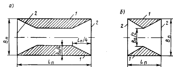
Рис. 1.2.6.3.1 Районы подкрепления и/или компенсации больших вырезов в стенках рамных балок днищвого набора:
