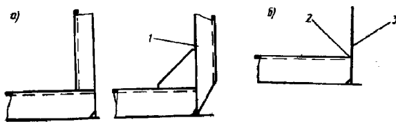
Рис. 2.2.3.1.3 Окончание продольных балок: 1 — вариант; 2 — см. 1.1.12; 3 — проникающая конструкция
