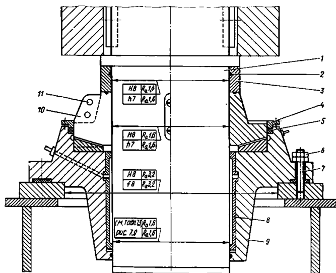
Рис. 1.1-5 Опорно-упорный подшипник баллера:
