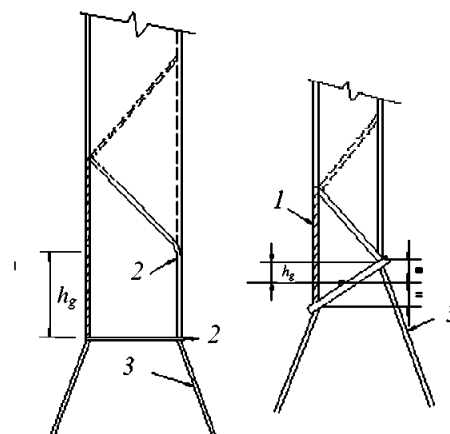
Рис. 1.4.2-4 Несимметричные гассетный/шедерные листы: 1 — гассетный/шедерный лист; 2 — горизонтальный/наклонный лист опоры (полки) нижней опоры для переборки; 3 — вертикальная/наклонная стенка нижней опоры для переборки
