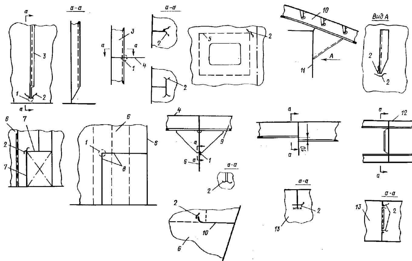
Рис. 1.1.12-1 Жесткие точки:
