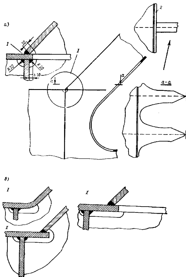
Рис. 2.2.3.10.2 Соединение настила второго дна с обшивкой наклонной стенки скуловой цистерны:
