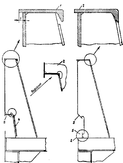
Рис. 2.7.9.4.2 Подкрепление кромки обшивки фальшборта у сплошной прозеи:
