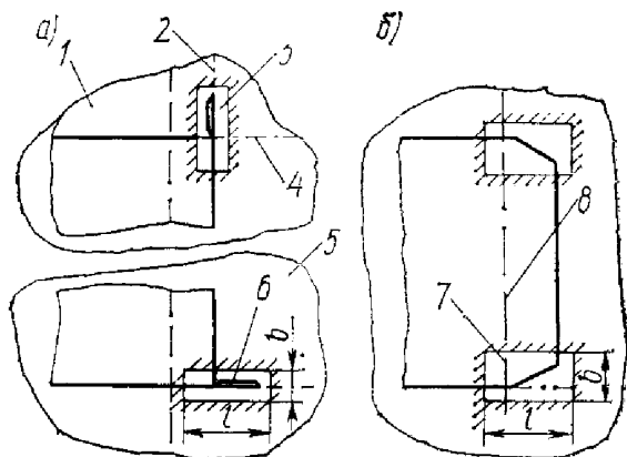
Рис. 2.7.2.5 Соединения боковых стенок рубок с концевыми переборками:
