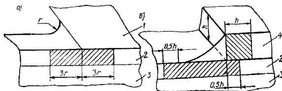
Рис. 1.4.3.7 Особые участки подкреплений вырезов в ширестреке:
