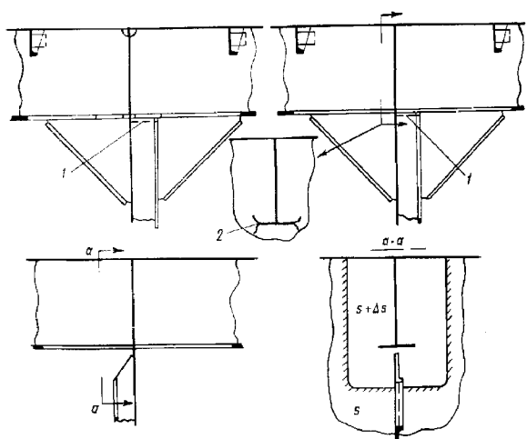
Рис. 2.4.4.1 Соединения карлингсов с поперечными переборками: 1 — вариант; 2 — см. 1.1.12
