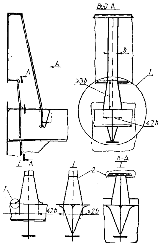
Рис. 2.7.9.5.4 Усиление стойки фальшборта:
