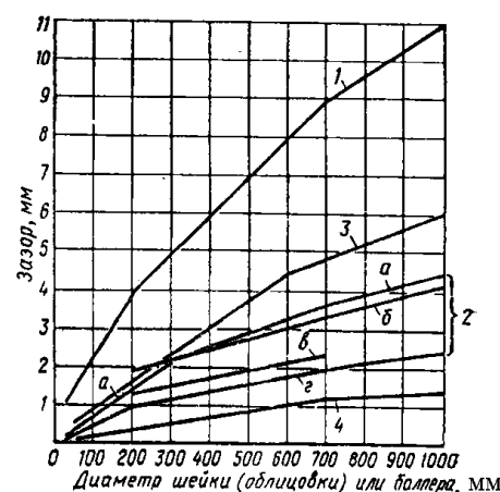
Рис. 3.2 График для определения зазоров в подшипниках пера руля (поворотной насадки) и баллера:
