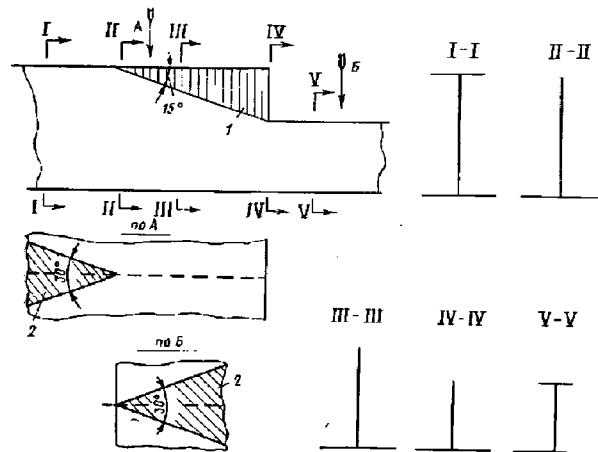
Рис. 2.2.3.8.1 Неэффективные участки флора в районе уступа двойного дна:
