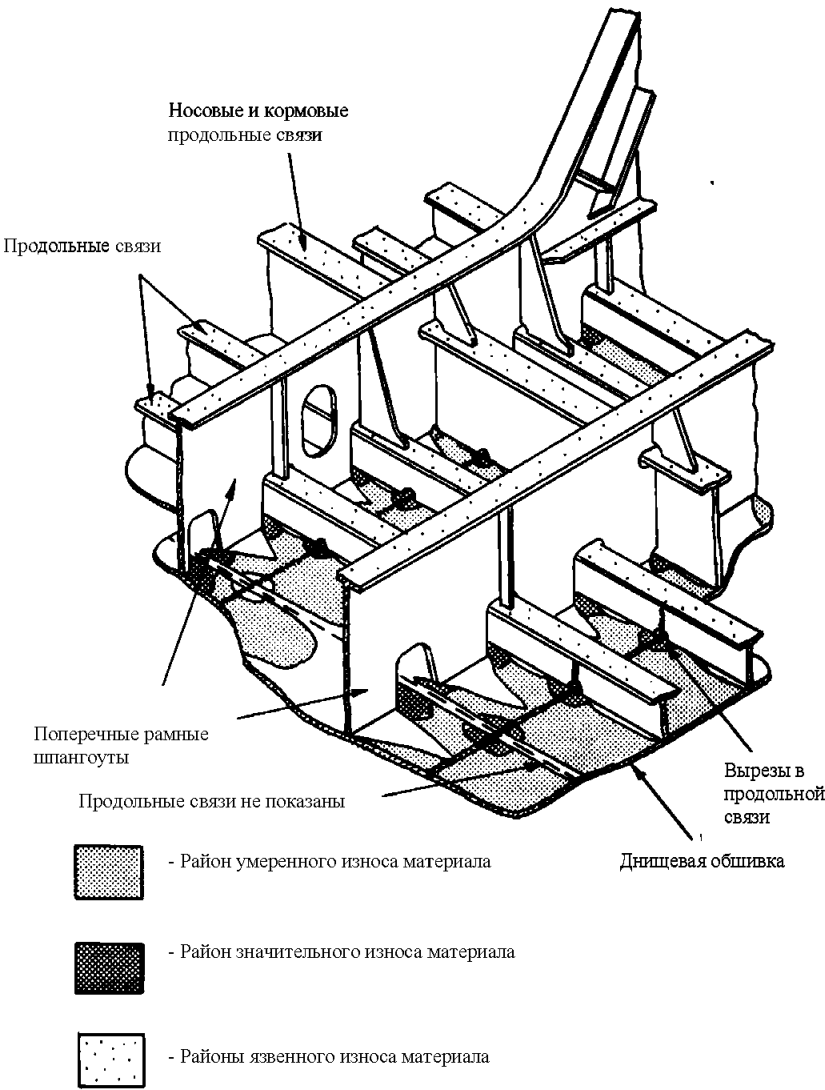
Рис. 6-1 Элементы корпусных конструкций танкеров, наиболее подверженные коррозионному износу
