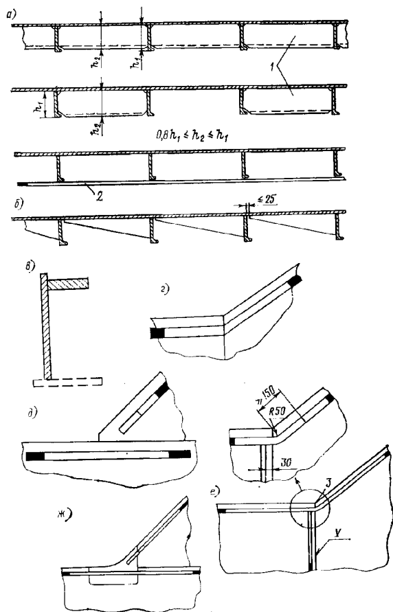
Рис. 1.2.2.4 Подкрепление, препятствующее закручиванию несимметричных профилей, и узлы их соединения:
