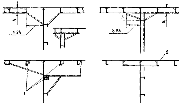
Рис. 2.3.6.2 Соединения стрингеров с поперечными переборками: 1 — заделки; 2 — правильно
