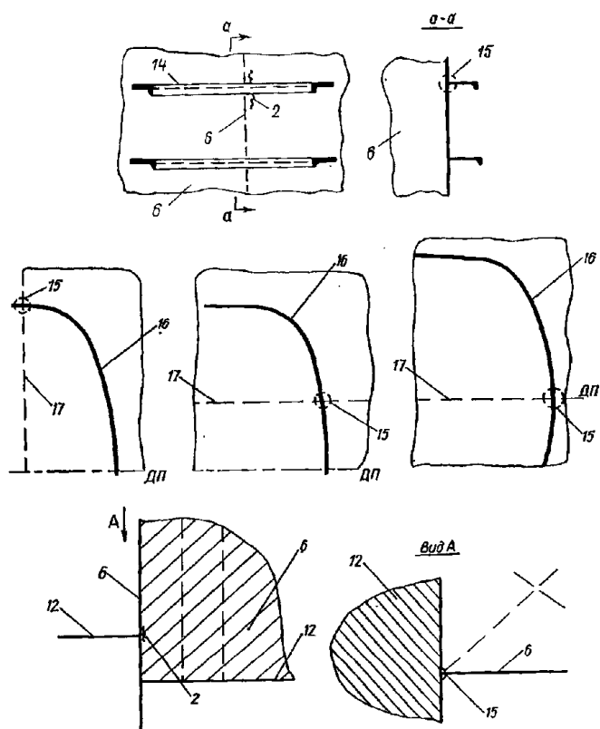
Рис. 1.1.12-2 Ножевые опоры:
