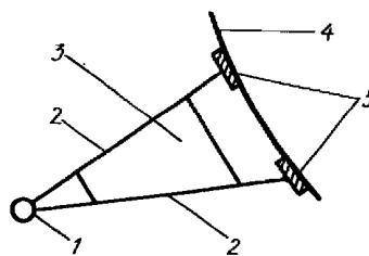
Рис. 2.1.5.2 Полый скуловой киль с двойными листовыми элементами:
