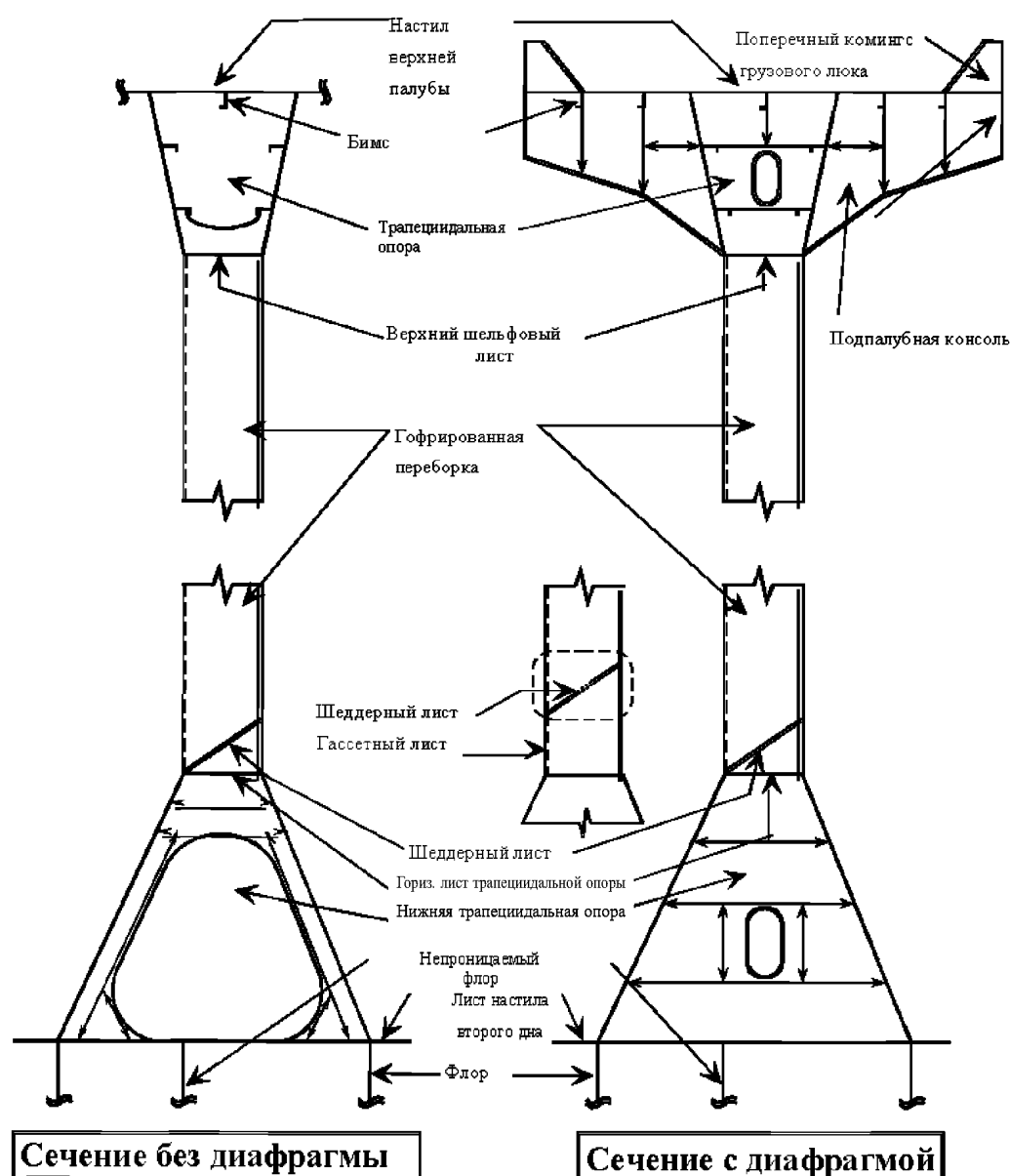
Рис. 2.2.1-2 Типичная водонепроницаемая переборка балкера
