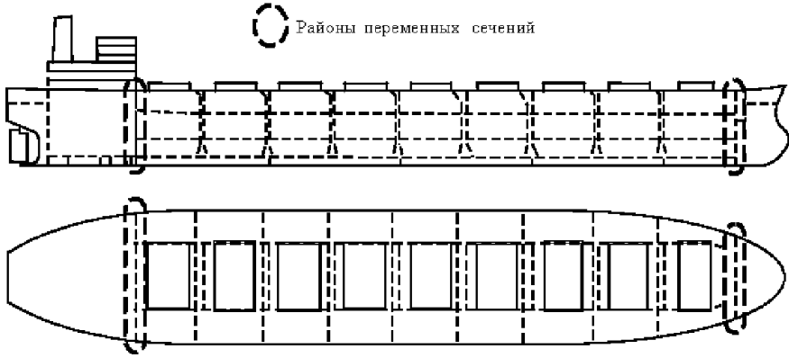
Рис. 4.3-3 Районы переменных сечений — Участки возможных повреждений
