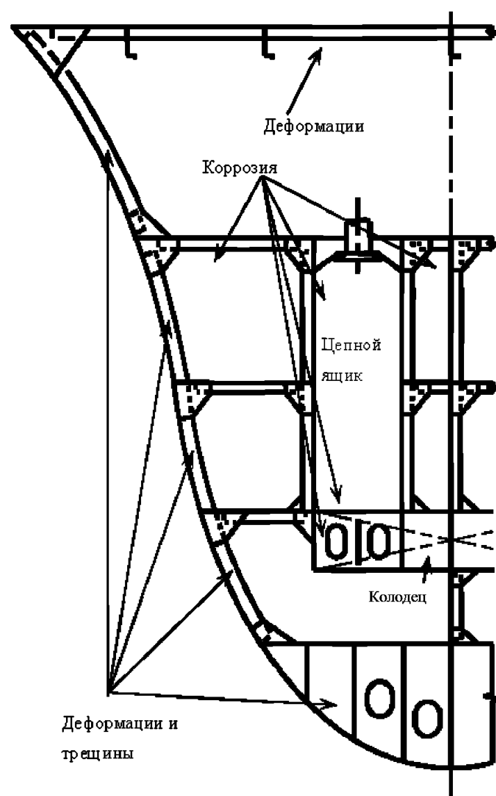
Рис. 3.2.1 Конструкция носовой оконечности — Участки возможных повреждений
