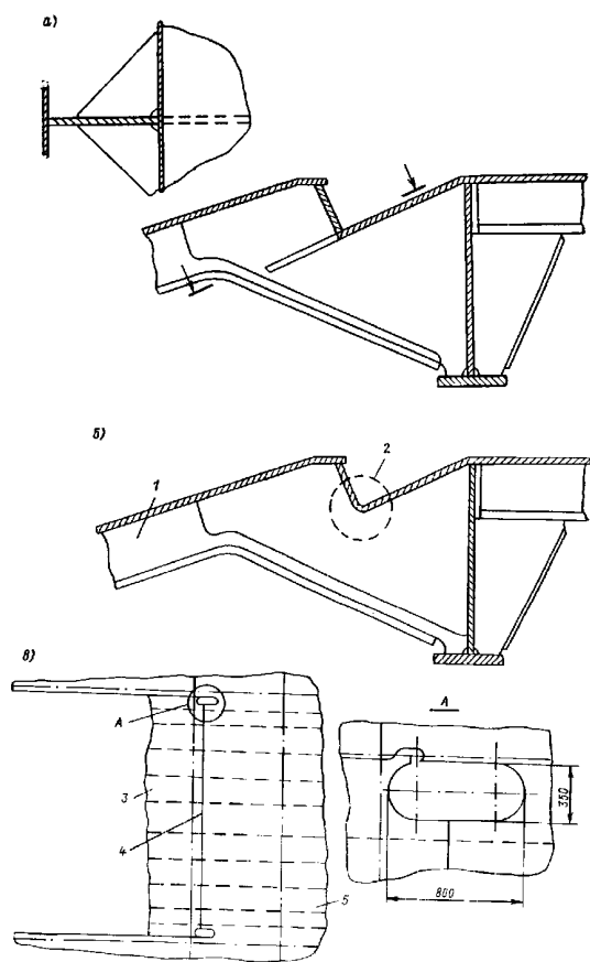
Рис. 2.4.18.3 Узел соединения съездной ramпы с палубой (а), скругление настила палубы по дуге малого радиуса (б) и переход настила верхней палубы (второго дна) в настил наклонного съезда (в):
