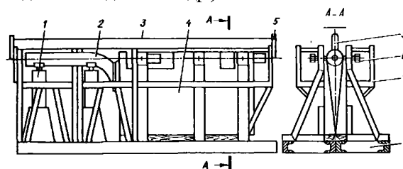
Рис. 5.2-1 Универсальный стенд для проверки соосности баллера пера руля:
