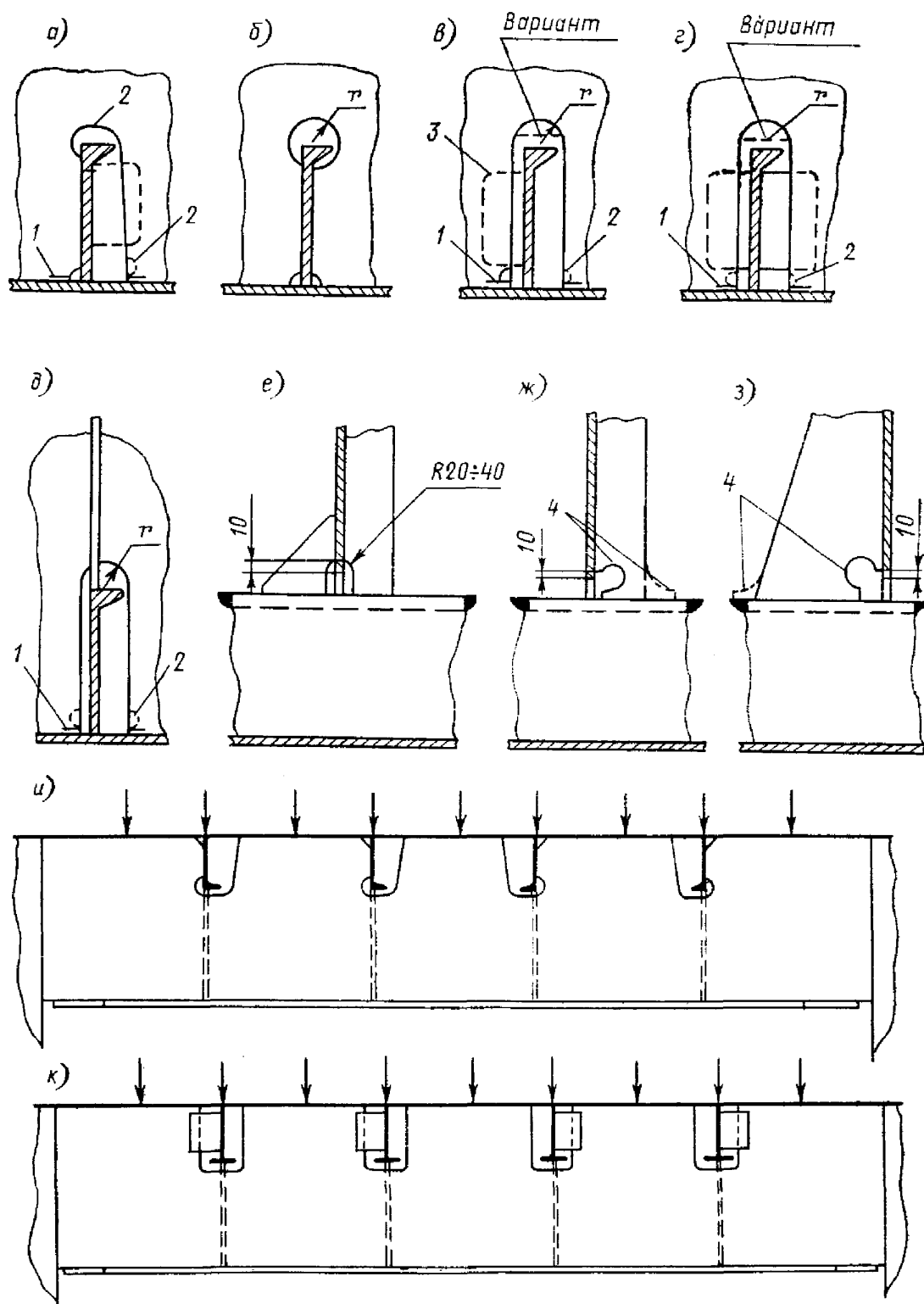
Рис. 1.3.4.2 Узлы соединения балок основного набора с поддерживающими их балками рамного набора:
