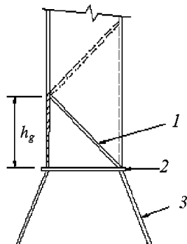
Рис. 1.4.2-2 Несимметричные шедерные листы: 1 — шедерный лист; 2 — горизонтальный/наклонный лист опоры (полки) нижней опоры для переборки; 3 — вертикальная/наклонная опорная стенка нижней опоры для переборки
