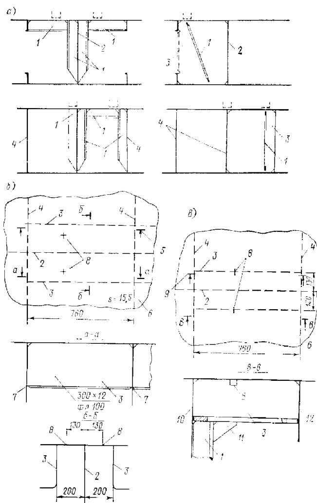
Рис. 2.2.3.10.1 Подкрепления двойного дна при перевозке контейнеров:
