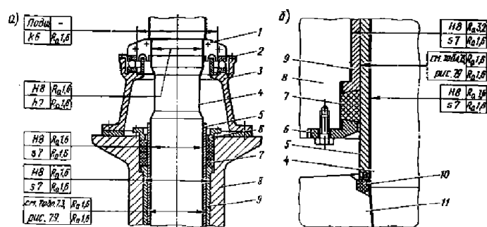
Рис. 1.1-2 Верхний (а) и нижний (б) гильпортовые подшипники баллера:
