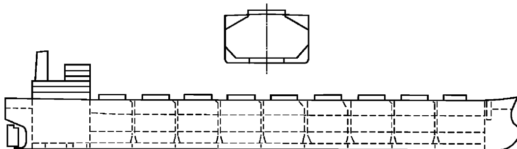
Рис. 1-1 Общий вид типичного балкера с одинарной обшивкой
