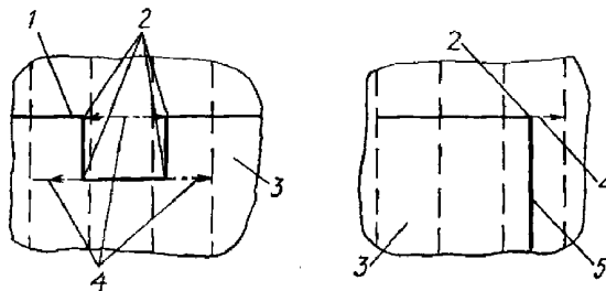
Рис. 2.4.13.3 Установка подкреплений для исключения жестких точек:
