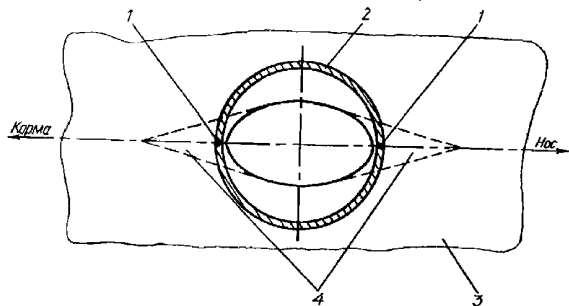
Рис. 1.4.2.6.3 Расположение стыковых швов в районах круглых (эллиптических) вырезов:
