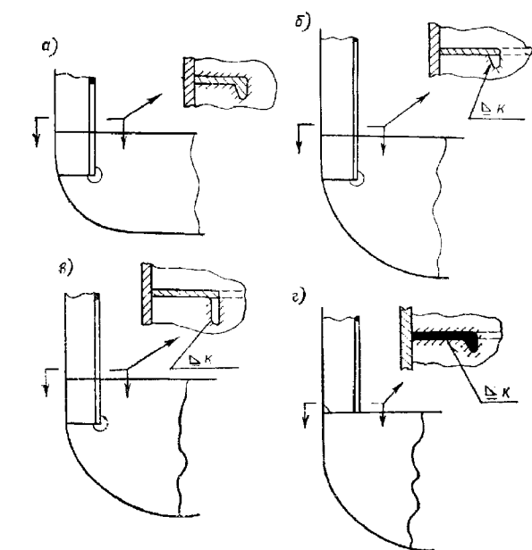
Рис. 2.3.1.4 Бесконечные соединения шпангоута с двойным дном: а — правильно; б — неправильно (площадь сечения бульба или пояска замаскируется площадью сварного шва, обваривающего профиль по периметру поперечного сечения); в — неправильно; г — неправильно (бульб обрывается у настила второго дна)
