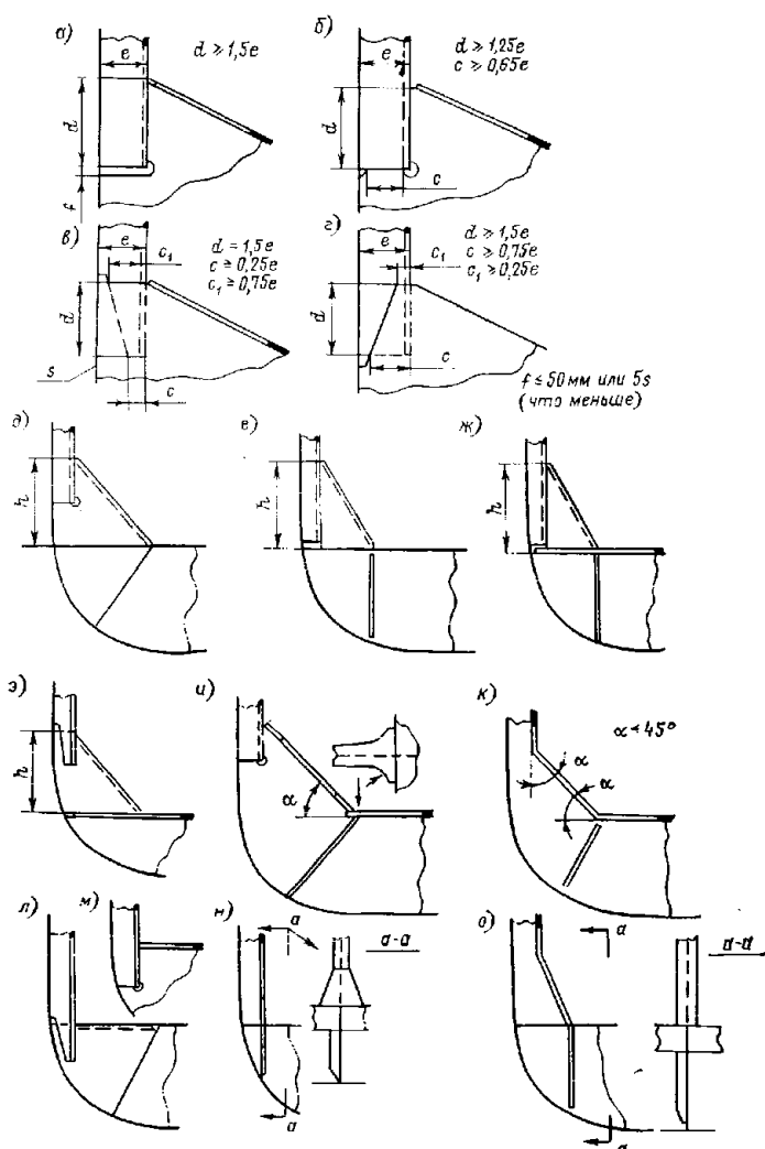
Рис. 2.3.1.1 Соединения нижнего конца шпангоута с днищевым набором
