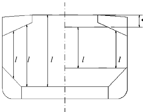
Рис. 1.3.1 Определение пролета гофра:
