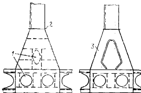
Рис. 2.2.3.10.4 Конструкция соединения трапецидальной опоры с двойным дном:
