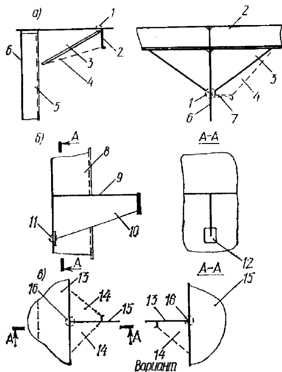
Рис. 1.1.13 Исключение жестких точек (а), смягчение жестких точек при ремонте (б) и исключение пожевых опор (в):
