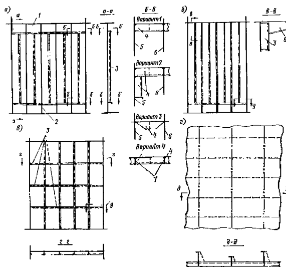
Рис. 2.9.1.6 Подкрепления листов обшивки (настила): 1 — продольная переборка; 2 — флор; 3 — дополнительная (промежуточная) балка набора; 4 — ребро жесткости; 5 — переборка; 6 — флор; 7 — балка набора; 8 — бракета; 9 — применить по б
