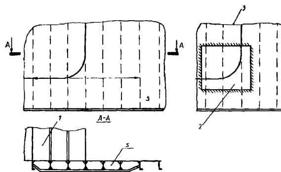
Рис. 2.4.13.2 Подкрепления у концевых переборок рубок: 1 — продольная стенка рубки; 2 — угольный сварной лист; 3 — неправильно
