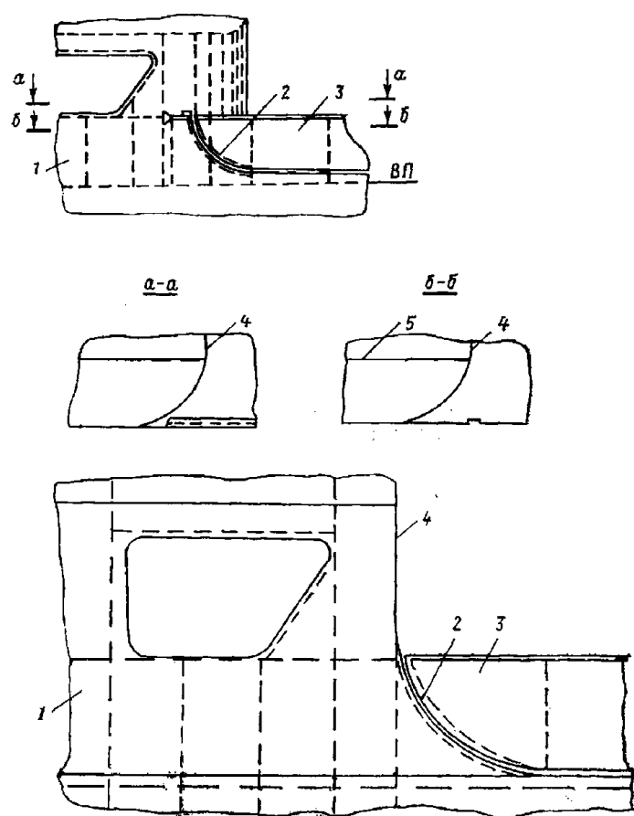
Рис. 2.7.4.3.3 Конструкция перехода выступающего листа обшивки прочных декоративных стенок в фальшборт:
