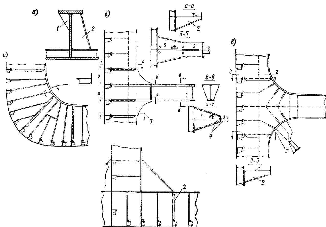
Рис. 1.2.3.3 Установка knees устойчивости:
