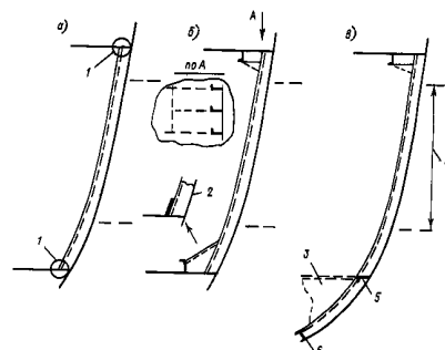
Рис. 2.3.3.3 Закрепление концов промежуточных шпангоутов:
