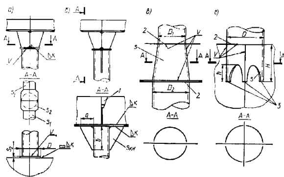
Рис. 2.4.8.1 Конструкции закрепления верхних и нижних концов пиллерсов:
