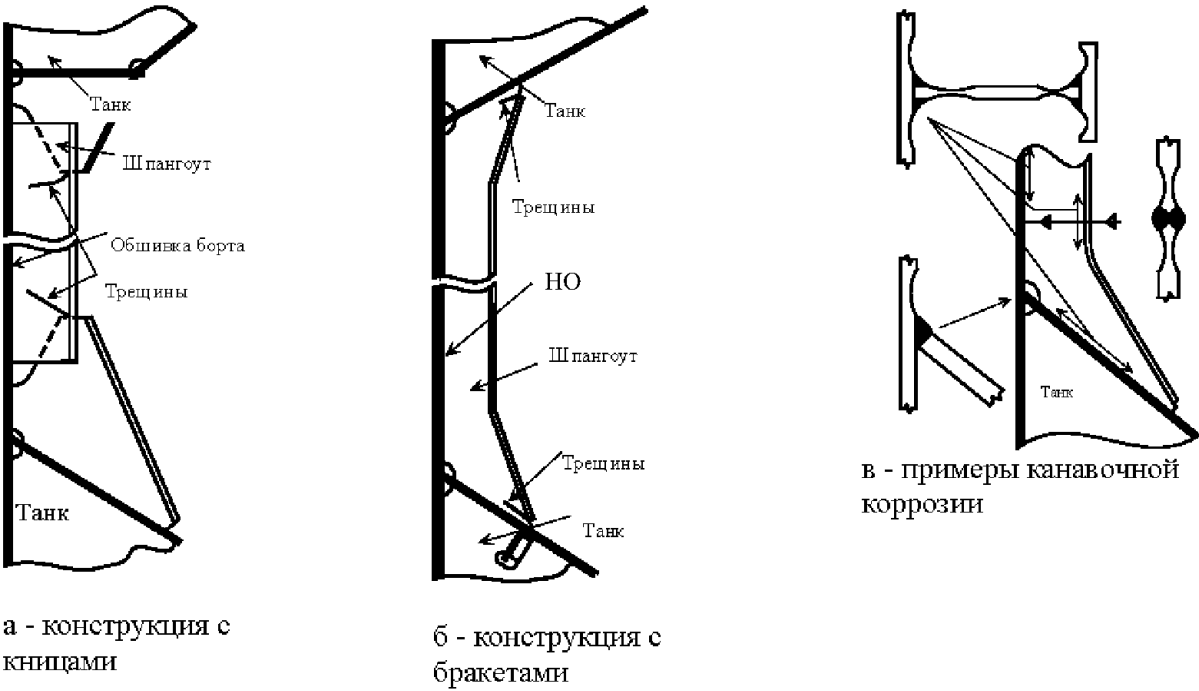
Рис. 4.3-2 Шпангоут — Потенциально проблемные участки
