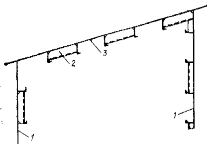
Рис. 2.9.1.4 Попарная перевязка рядом расположенных балок набора: 1 — переборка; 2 — бракета с фланцем или профиль; 3 — борт
