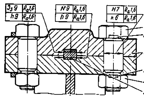
Рис. 1.1-4 Фланцевое соединение баллера или съемного рудерпоста:
