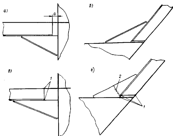
Рис. 2.9.1.8 Закрепление кницами концов балок и пиллерсов:
