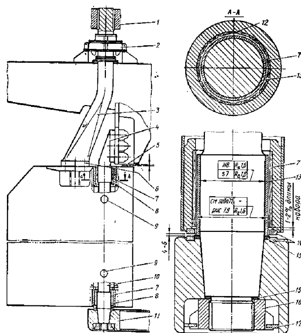
Рис. 1.1-3 Рулевое устройство со съемным рудерпостом:
