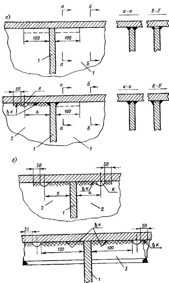
Рис. 1.3.4.20 Перемычки в местах прохода балок основного набора через стенки непроницаемых конструкций:
