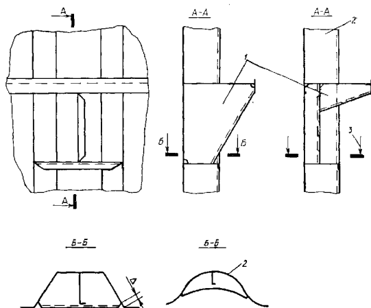
Рис. 2.5.4.5 Закрепление концов книц устойчивости на переборке:
