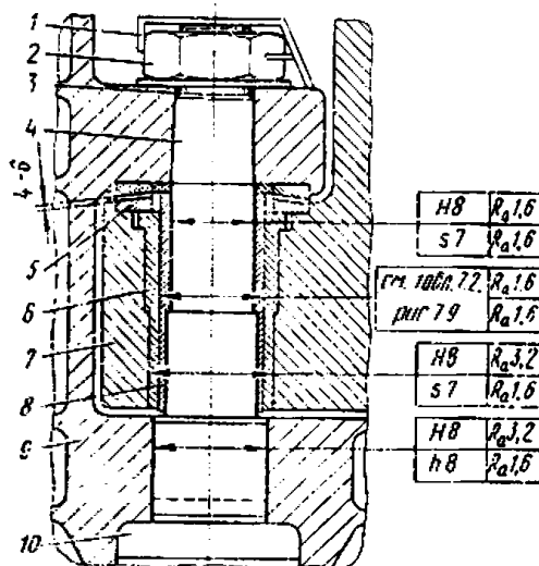
Рис. 1.1-6 Штырь с цилиндрической направляющей втулкой:
