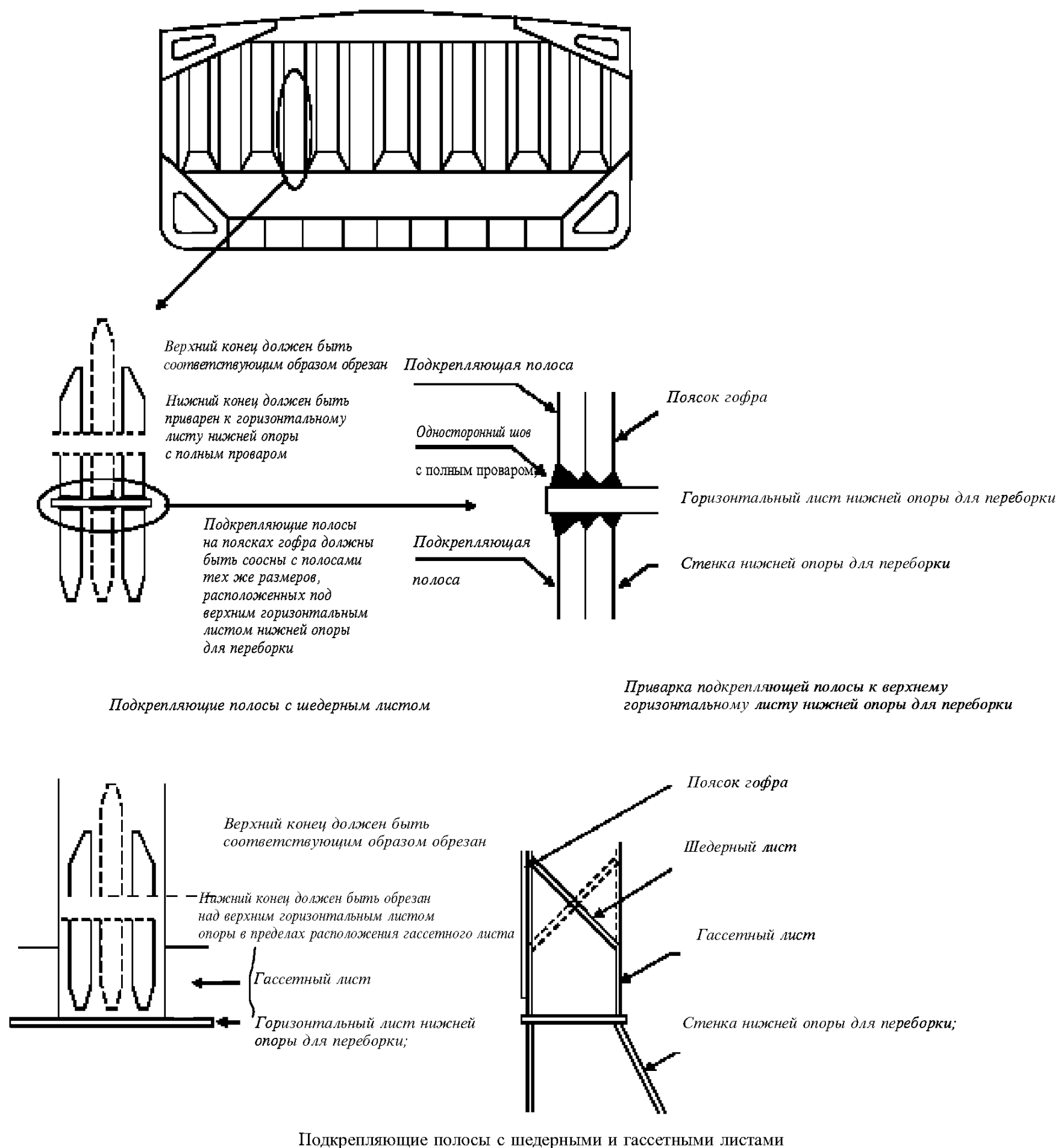
Рис. 2.6 Общая схема гофров переборки
