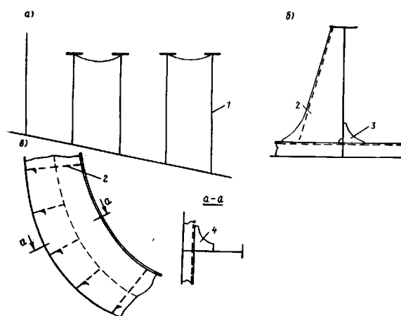
Рис. 2.9.1.5 Увеличение жесткости рамных балок в направлении, перпендикулярном к плоскости их стенки: 1 — флор; 2 — кница устойчивости; 3 — смягчающая кница; 4 — кница
