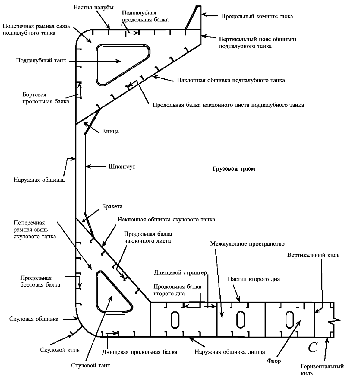
Рис. 2.2.1-1 Типичный поперечный разрез грузового трюма балкера
