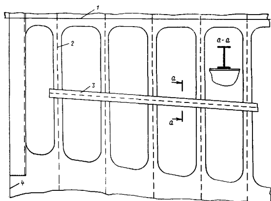
Рис. 2.9.2.9 Увеличение жесткости флоров в направлении вдоль судна:
