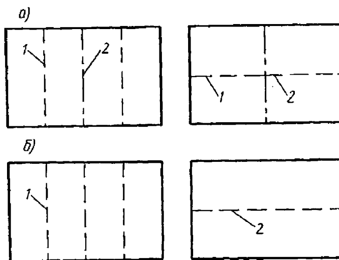
Рис. 2.2.3.5.3 Подкрепление стенок вертикального киля (а) и днищевого стрингера (б): 1 — ребро жесткости; 2 — бракета
