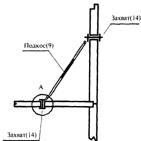
Схема 1а
