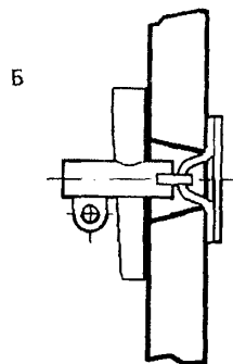
Рисунок 5 – Временное крепление наружных панелей
