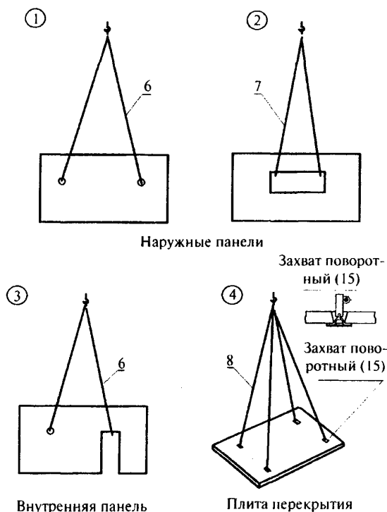
Рисунок 2 – Схемы строповки
