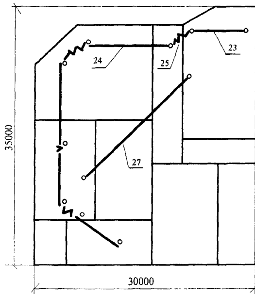
Рисунок 9 – Схема расположения ограждения опасной зоны и страховочных приспособлений
