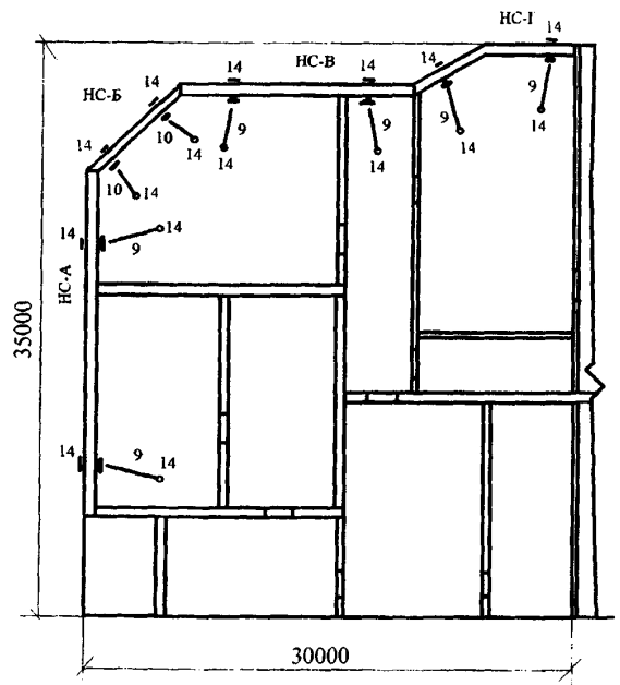
Рисунок 7 – Схема временного крепления наружных панелей
