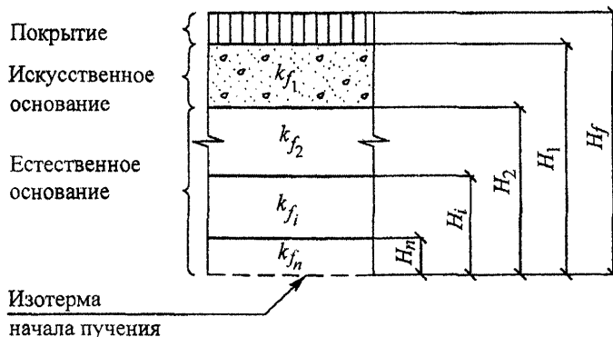
Рисунок Е.1 – Расчетная схема слоистого основания
