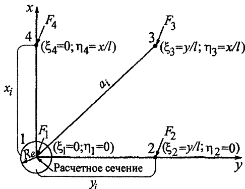
Рисунок 7.2 – Расчетная схема параметров загрузки опор воздушного судна
