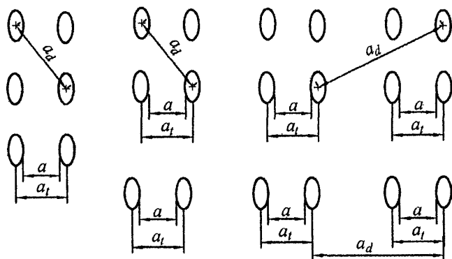
Рисунок К.7 – Расчетные расстояния a, a_n, a_d между колесами опор воздушных судов
