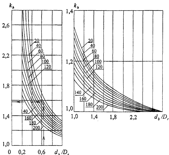
Рисунок Г.1 – График для определения коэффициента k_h жесткого массива. Цифрами на кривых указан коэффициент постели слоя основания K_{sr} , \text{МН/м}^3 , лежащего на жестком массиве
