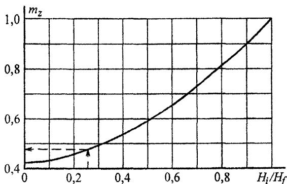
Рисунок Е.2 – График для определения коэффициента m_z
