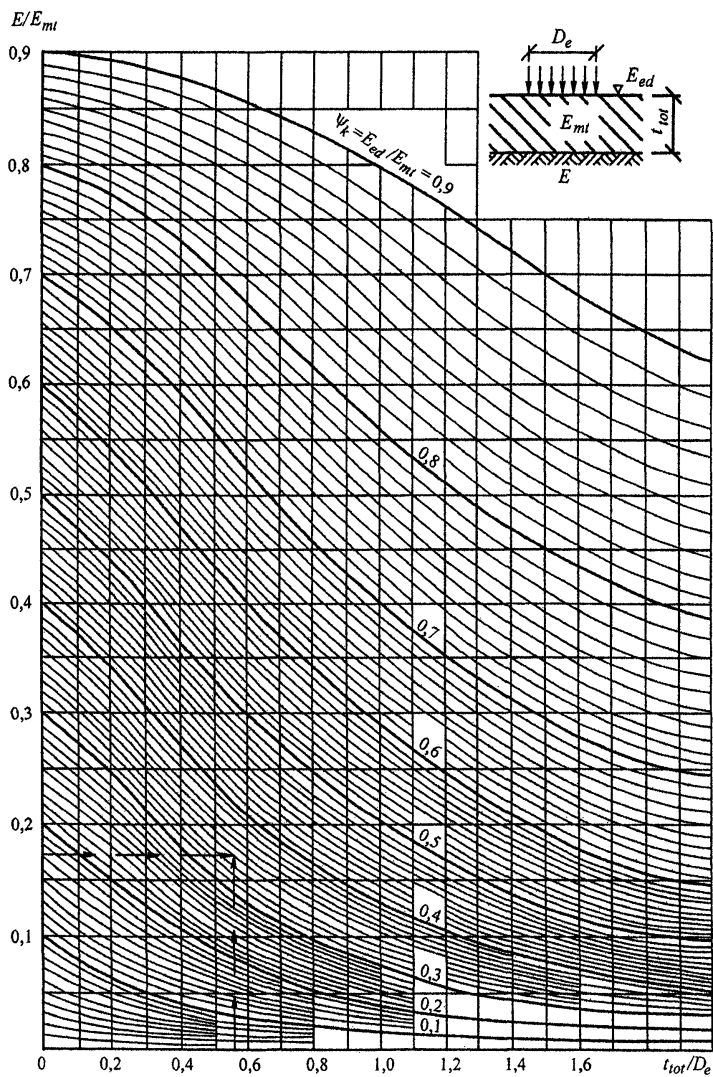
Рисунок К.4 – Номограмма для определения коэффициента \Psi_k
