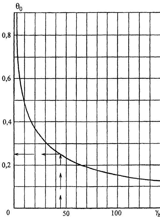
Рисунок М.1 – График для определения \theta_0
