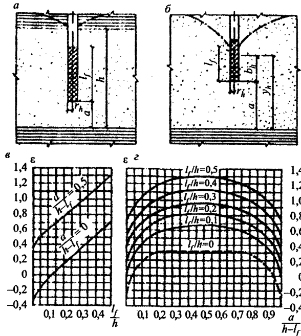
а, б – схемы несовершенных скважин в напорном и безнапорном пластах; в, з – графики для определения \varepsilon
