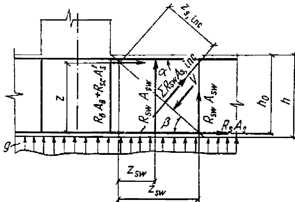
Рисунок Г.7 – Схема усилий в сечении, наклонном к продольной оси железобетонного элемента, при расчете его по прочности на действие изгибающего момента
