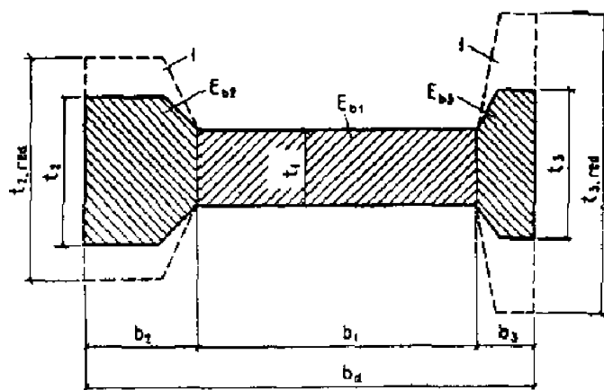
1 – контур приведенных сечений оголовков в случае приведения их модулей упругости бетона E_{b2} и E_{b3} к модулю упругости бетона контрфорса E_{b1} (при E_{b3} > E_{b2} > E_{b1} )
