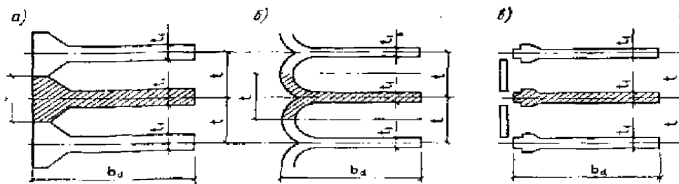
а – для массивно-контрфорсных плотин; б – для плотин с неразрезным арочным перекрытием; в – для плотин с разрезным напорным перекрытием; t_1 – толщина контрфорса; t – длина секции; b_d – ширина расчетного сечения
