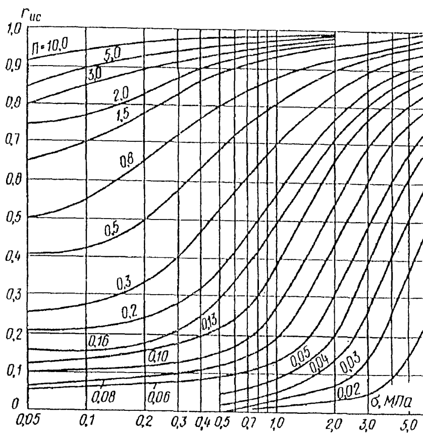
Рисунок Б.3.1 — Номограмма для определения порового давления r_{ис} .
