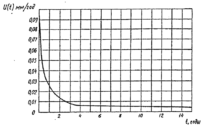
Рисунок В.12.5 — Изменение средней скорости коррозии стальной диафрагмы в водно-грунтовой среде Северной строительно-климатической зоны
