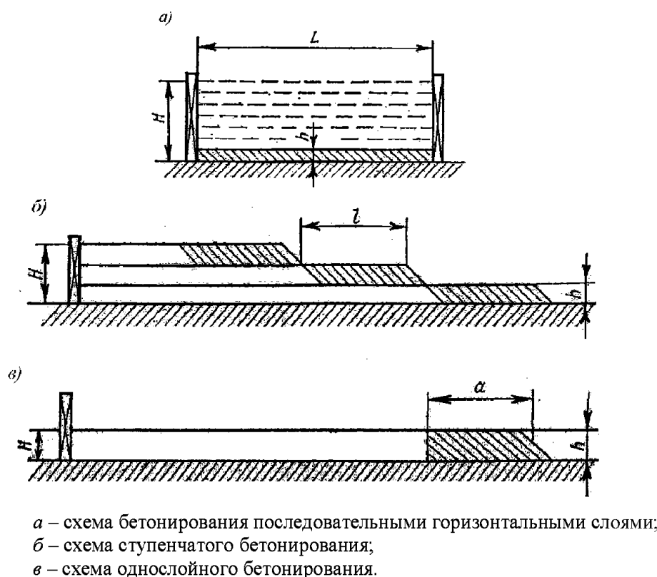
Рисунок Е.1 – Основные схемы укладки бетонной смеси в блоки
