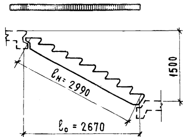
Расчетная схема
