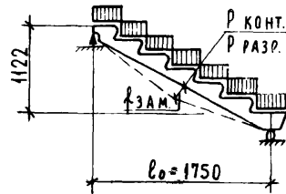
Схема загрузки при испытании
