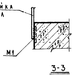
Деталь крепления перила на сварке
