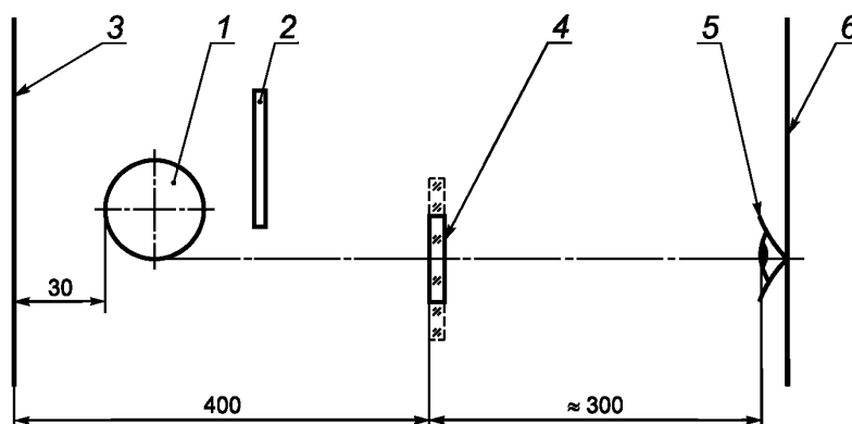
1 — источник света (люминесцентная лампа); 2 — регулируемая черная непрозрачная маска; 3 — черный матовый экран; 4 — испытываемая очковая линза; 5 — глаз испытателя; 6 — плоскость наблюдения
