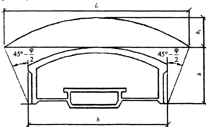
Рисунок 5.1 – Схема для расчета высоты свода обрушения
