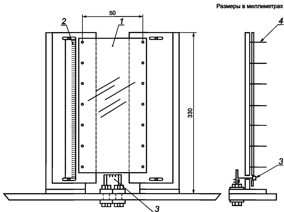
1 — образец; 2 — шкала; 3 — источник воспламенения; 4 — игла
