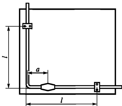
Рисунок D.2 — Конфигурация проводников в LPS
