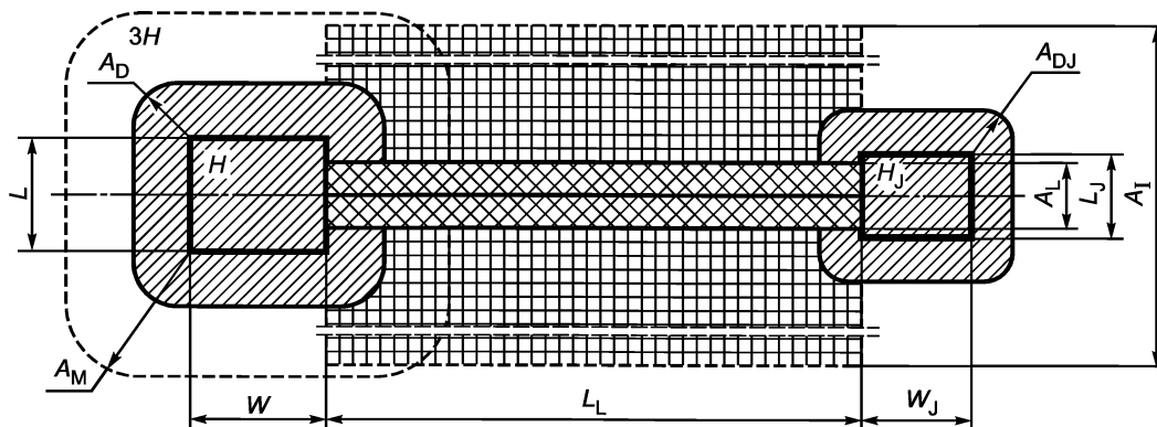
Рисунок A.5 — Области защиты (область покрытия) ( A_D , A_M , A_I , A_L )
