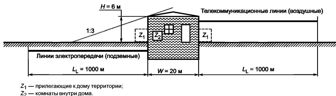
Рисунок Е.1 — Дом в сельской местности
