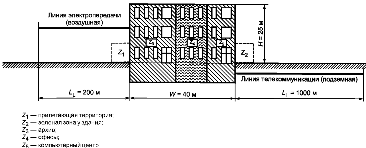
Рисунок Е.2 — Административное здание
