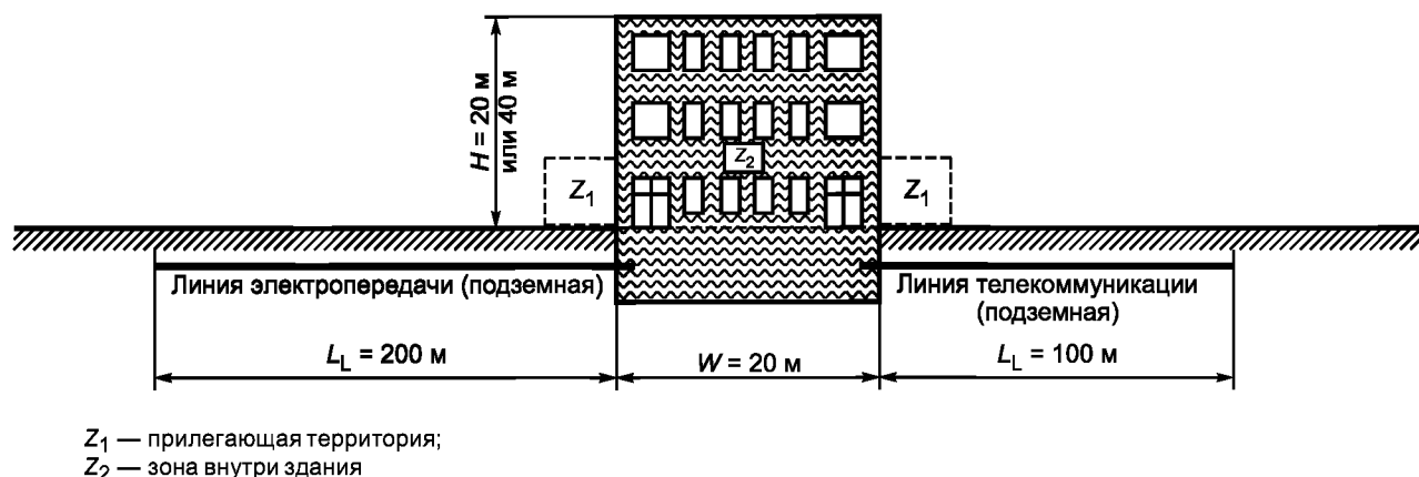
Рисунок Е.4 — Жилой дом
