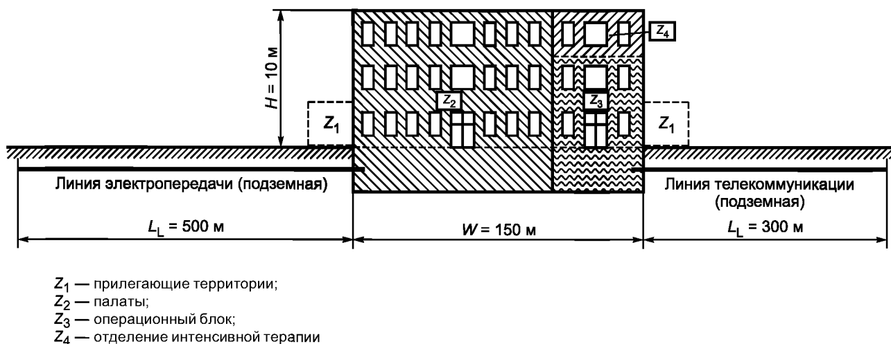
Рисунок Е.3 — Больница
