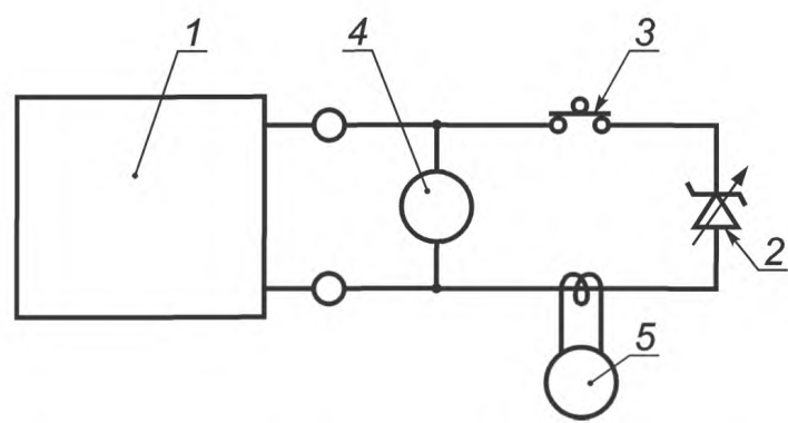
1 — испытываемая цепь; 2 — нагрузка; 3 — ртутный выключатель; 4 — вольтметр высокого сопротивления; 5 — щуп для замера величины тока
