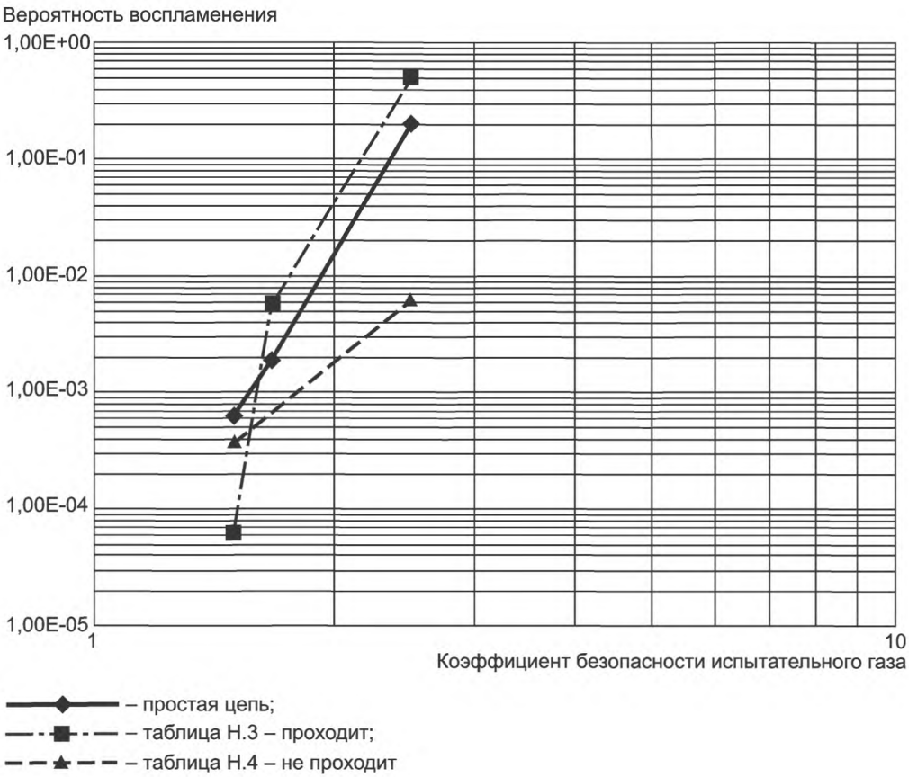
Рисунок Н.1 — Кoeffициент безопасности в зависимости от вероятности воспламенения
