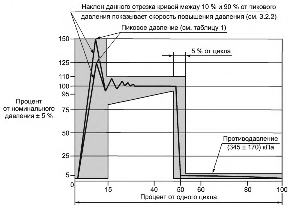
Рисунок — Кривая импульса
