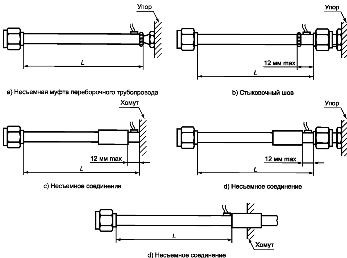
Рисунок 3 — Способы установки образцов с несъемной муфтой
