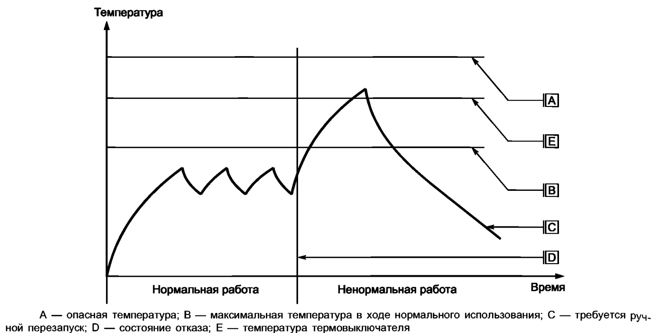
Рисунок ЕЕ.5 — Термовыключатель без самовозврата
