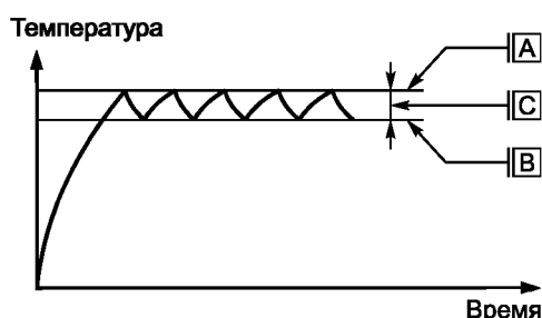
Рисунок ЕЕ.1 — Терморегулятор
