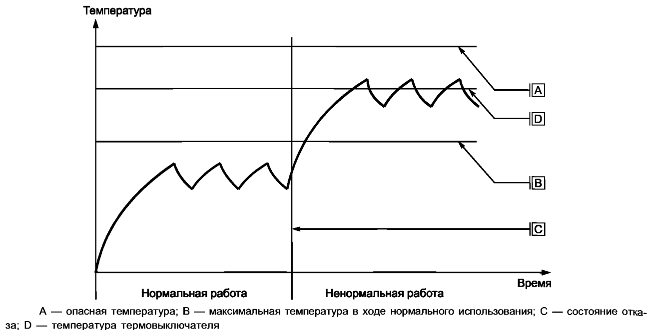
Рисунок ЕЕ.4 — Термовыключатель с самовозвратом
