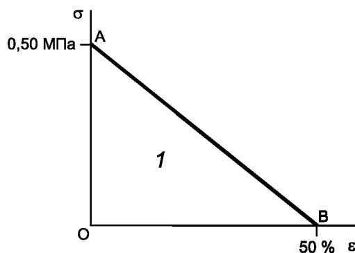
Рисунок 1 — Треугольник зависимости напряжений от деформации
