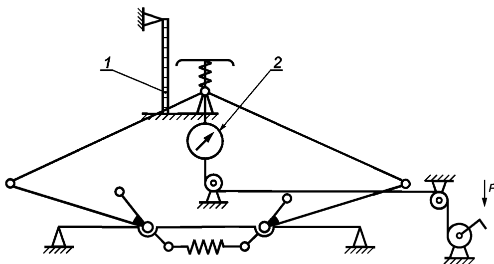
Рисунок 7 — Кинематическая схема для определения жесткости кареток
