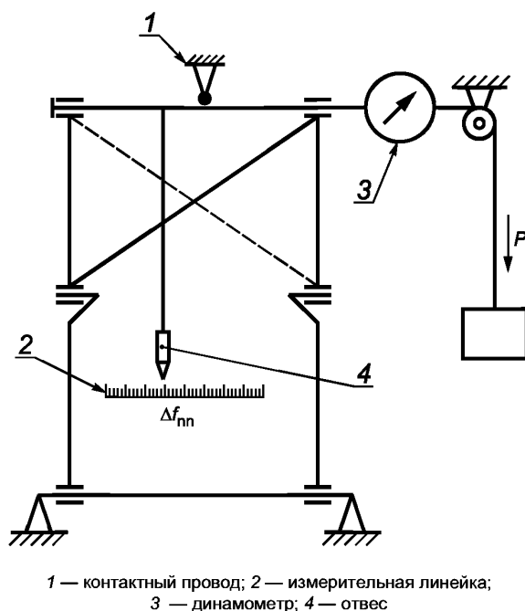
Рисунок 5 — Кинематическая схема для определения поперечной жесткости
