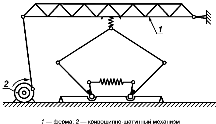
Рисунок 8 — Кинематическая схема колебательной установки
