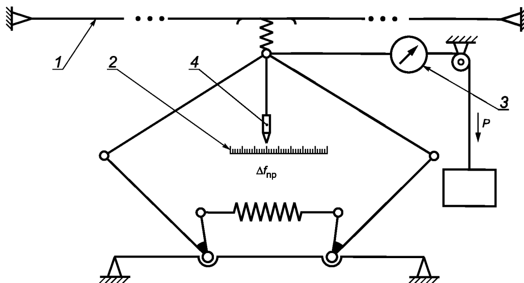
Рисунок 6 — Кинематическая схема для определения продольной жесткости
