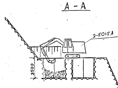
ПЕРЕМЕЩЕНИЕ ГРУНТА В ОТВАЛ
