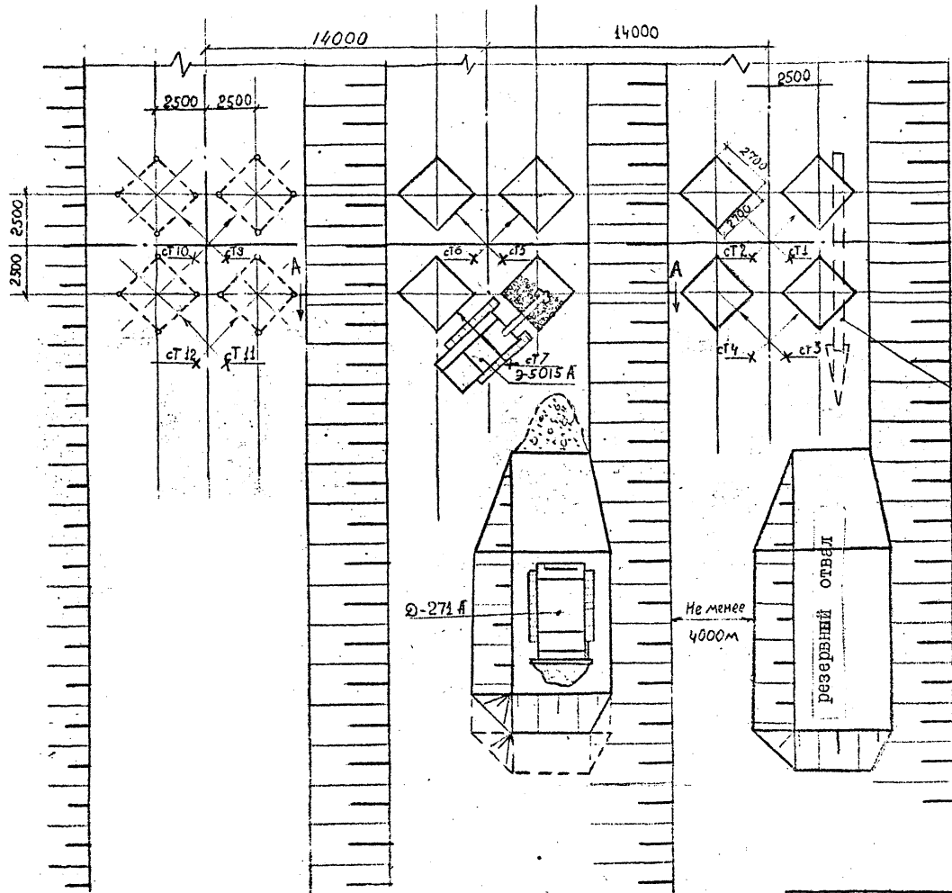
ПЕРЕМЕЩЕНИЕ ГРУНТА В ОТВАЛ
