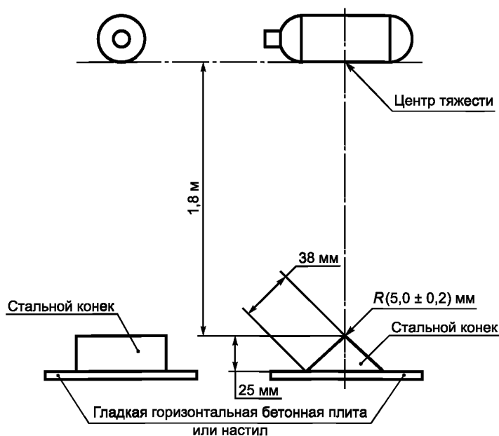
Рисунок 1 — Испытание контейнера падением на конек
