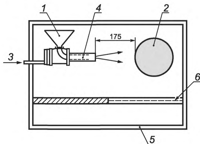
1 — воронка; 2 — испытываемая оболочка; 3 — впуск воздуха; 4 — труба \varnothing 50 \text{ мм} ; 5 — короб шириной около 500 мм; 6 — фильтр
