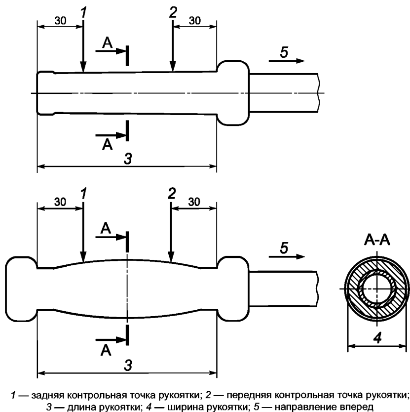
Рисунок 3 — Элементы рукоятки
