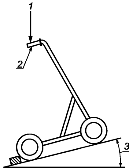
1 — нагрузка; 2 — задняя контрольная точка рукоятки; 3 — угол наклона
