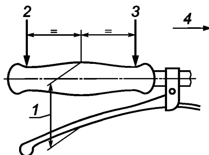
Рисунок 3 — Элементы рукоятки
