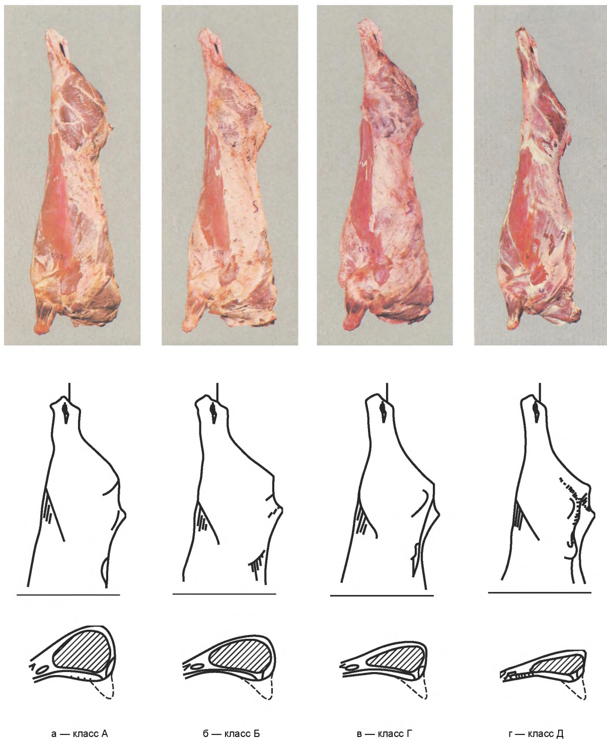
Рисунок 2 — Форма и полнотность туш по классам
