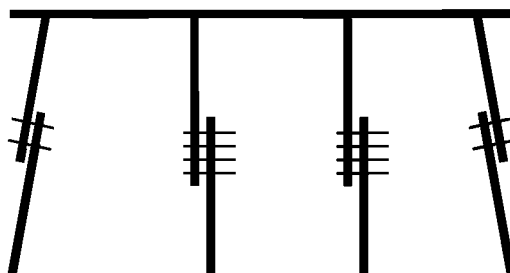
Рисунок 3 — Схема трапецевидной крепи с двумя дополнительными центральными стойками (боковые стойки могут быть криволинейными)
