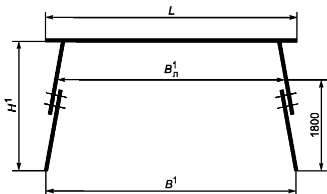
Рисунок 1 — Схема трапецевидной крепи (стойки могут быть криволинейными)
