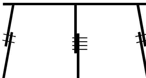
Рисунок 2 — Схема трапецевидной крепи с одной дополнительной центральной стойкой (боковые стойки могут быть криволинейными)
