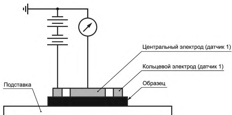
Рисунок 2 — Принцип подключения электродов для измерения поверхностного сопротивления
