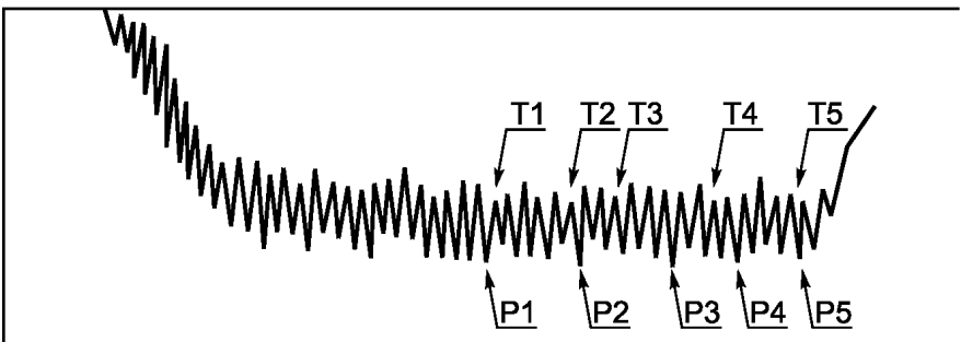
2б — Осциллограмма напряжения человеческого тела отрицательной полярности
