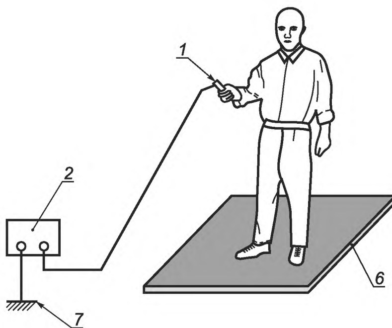
1б — Схема для испытаний установленных полов
