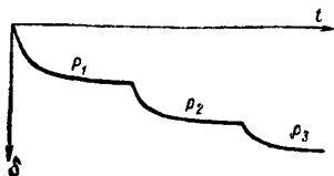
Рис. 12. Зависимость величины относительной деформации \delta от времени t при ступенчатом нагружении мерзлого грунта
