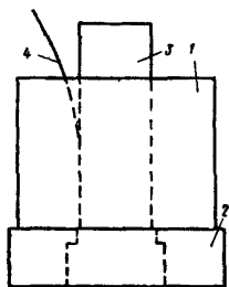
Рис. 38. Форма для замораживания образца грунта с моделью фундамента 1 — кольцо; 2 — поддон; 3 — модели фундамента; 4 — термопара
