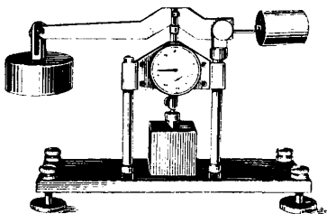
Рис. 19. Рычажный одноштоковый шариковый прибор конструкции Цытовича — Файнциммера
