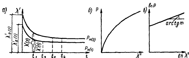
Рис. 24. Определение параметра m по данным испытаний
