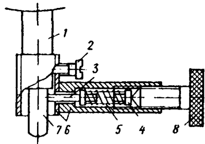
Рис. 28. Тормозное устройство
