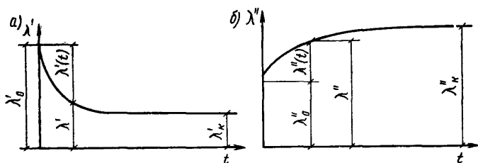
Рис. 23. Развитие деформаций во времени при испытаниях на динамометрическом приборе
