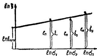
Рис. 40. Зависимость установившейся скорости относительной деформации от напряжения (в логарифмическом масштабе)
