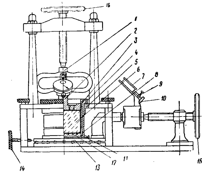
Рис. 27. Схема сдвигового прибора ВСВ-1
