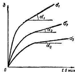
Рис. 39. Зависимость относительной деформации льда \delta от времени t при различных значениях напряжения ( \sigma_1 > \sigma_2 > \sigma_3 )
