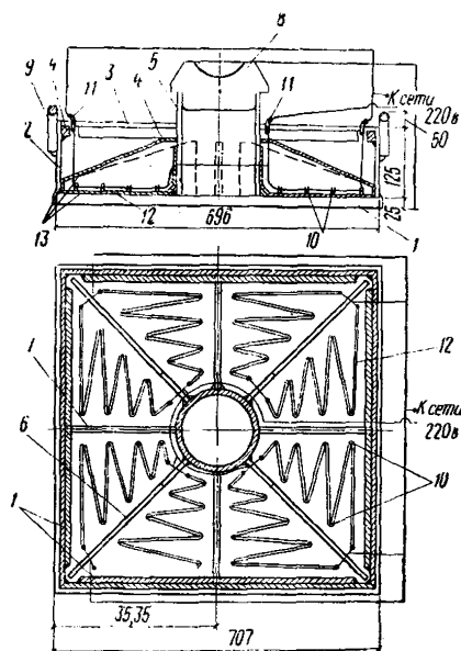
Рис. 14. Штамп с электрообогревом
