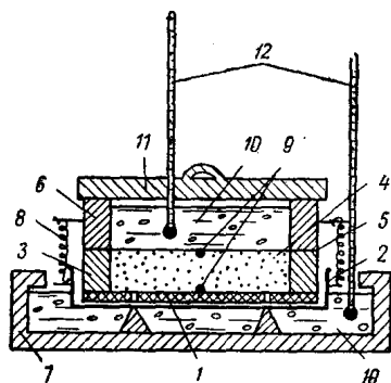
Рис. 8. Схема прибора для определения коэффициента теплопроводности мерзлых грунтов по методу стационарного теплового режима (упрощенный вариант)
