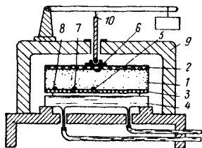
Рис. 7. Схема прибора для определения коэффициента теплопроводности мерзлых грунтов по методу стационарного теплового режима
