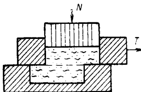
Рис. 25. Схема одноплоскостного сдвига
