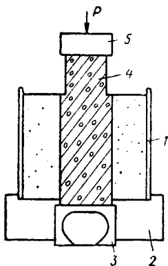
Рис. 31. Схема прибора Цытовича
