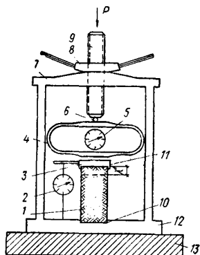
Рис. 22. Схема динамометрического прибора
