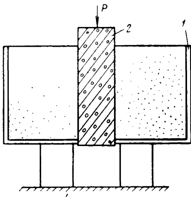
Рис. 32. Схема прибора Ермакова
