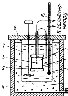
Рис. 10. Схема прибора для определения коэффициента теплопроводности грунта по методу регулярного теплового режима
