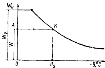
Рис. 2. Пример кривой зависимости содержания незамерзшей воды от отрицательной температуры и расчет температуры начала замерзания грунта
