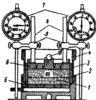
Рис. 11. Схема прибора для определения сжимаемости мерзлого грунта
