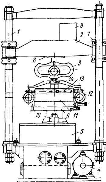
Рис. 37. Схема динамометрического пресса для определения сопротивления сдвигу мерзлого грунта по модели фундамента конструкции ЦНИИС Минтрансстроя
