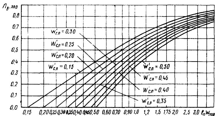
Рис. 6. Зависимость влажности горизонта мерзлого грунта W_{гор} от льдистости за счет ледяных включений, разделяющих слои, L_{в.гор} и средней влажности слоя W'_{сл}
