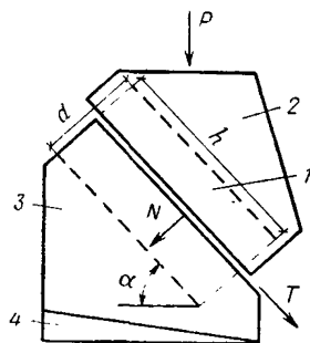
Рис. 26. Схема клинового прибора
