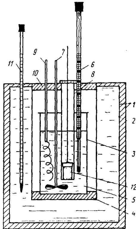
Рис. 4. Схема калориметра
