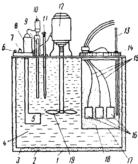
Рис. 3. Схема ультратермостата
