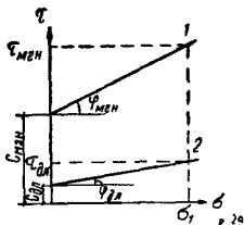
Рис. 29. Диаграммы сдвига
