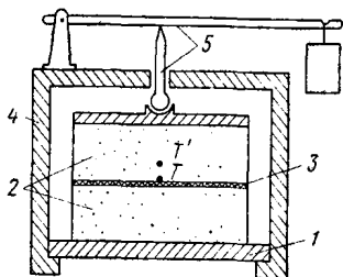
Рис. 9. Схема прибора для определения коэффициента теплопроводности грунтов по методу теплового импульса
