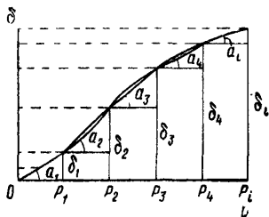
Рис. 13. Зависимость относительной деформации от давления p (компрессионная кривая)
