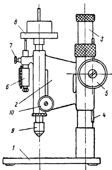
Рис. 18. Схема шарикового прибора (конструкция НИС «Гидропроекта»)
