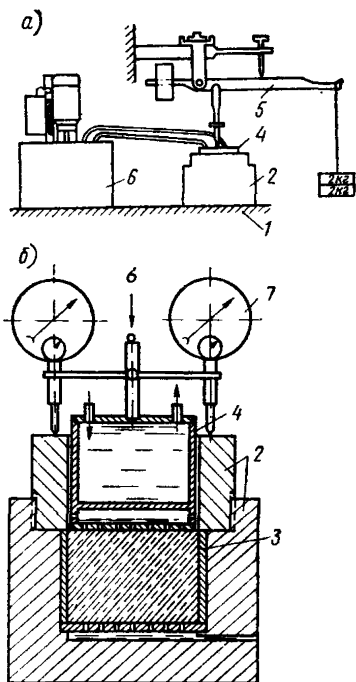
Рис. 16. Схема прибора для определения сжимаемости мерзлого грунта при оттаивании
