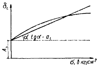
Рис. 17. Зависимость относительного сжатия \delta_i от давления \sigma_i
