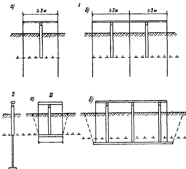
Рис. 36. Схемы анкерных опор
