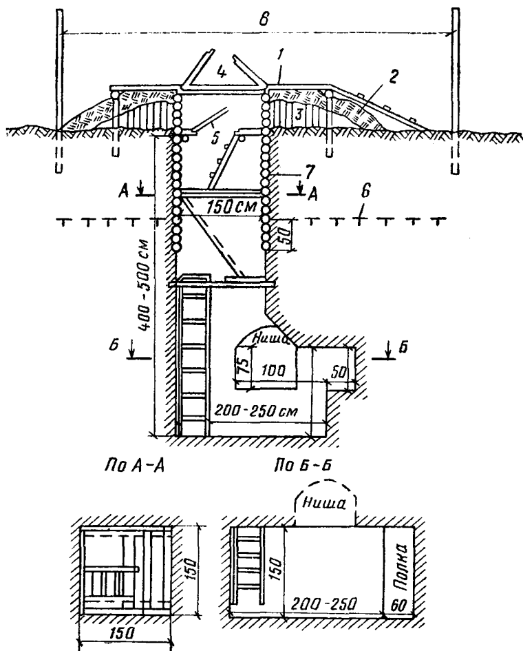
Рис. 1. Схема полевой лаборатории
