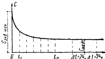
Рис. 21. Изменение во времени сопротивления мерзлого грунта вдавливаю шарикового штампа
