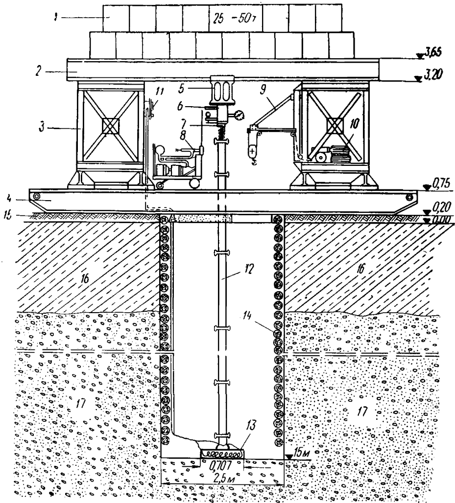
Рис. 15. Схема полевой установки для определения сжимаемости мерзлого грунта при оттаивании
