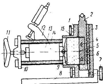
Рис. 33. Схема прибора НИИ оснований
