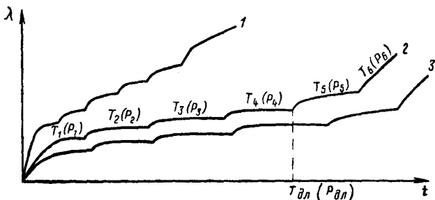
Рис. 30. Развитие деформаций во времени при нагружении ступенями
