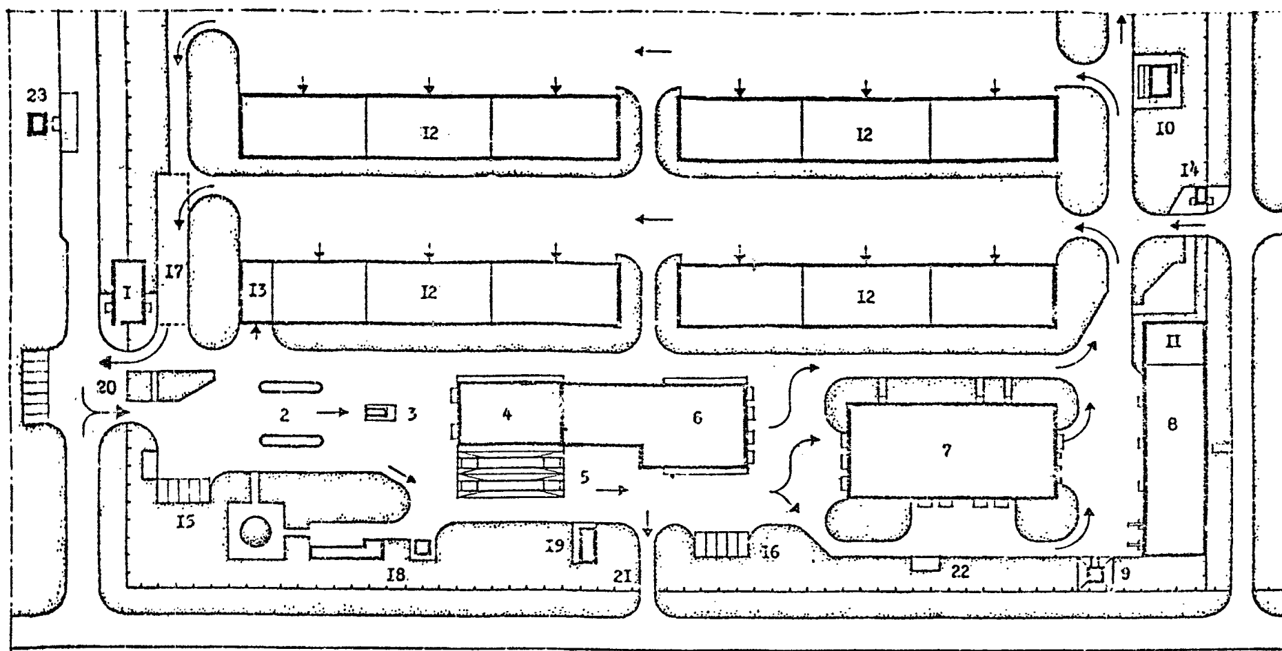
Рис. 3. Примерная схема технологической линии парка техники и вооружения (ТВ):
