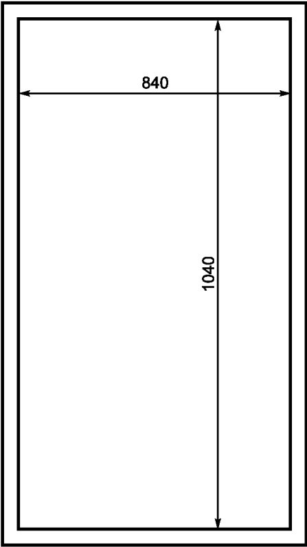
Изготовлено из стальных уголков 25 × 25 × 3 мм
