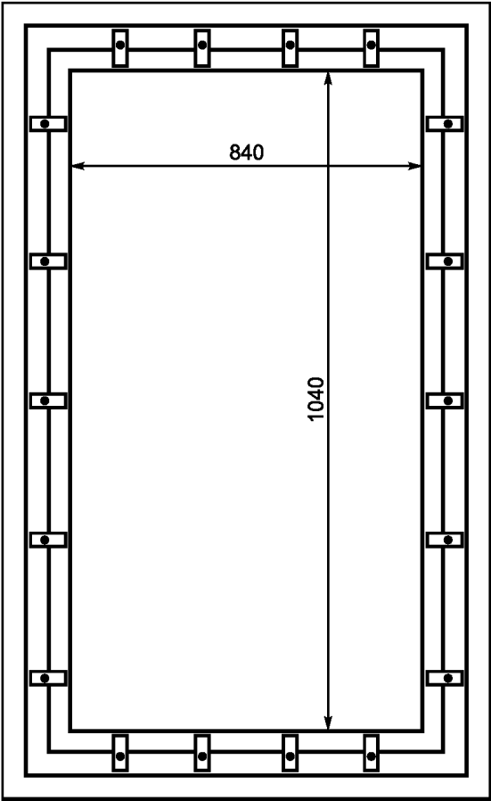
Изготовлено из стальной ленты 102 × 13 мм
