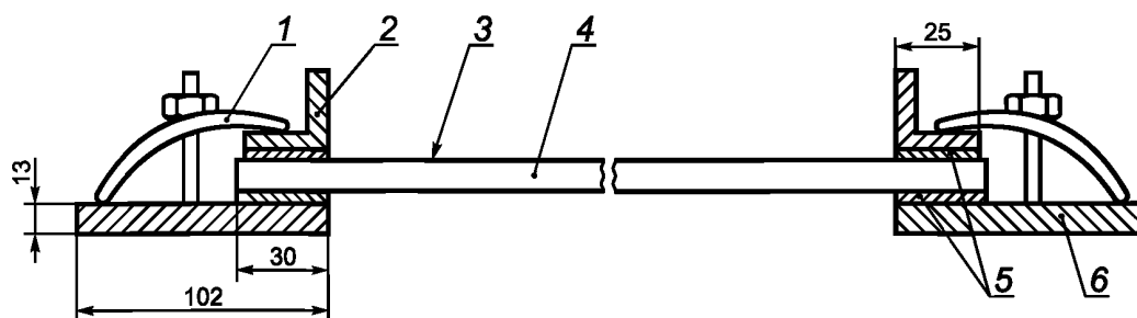
1 — зажим; 2 — внутренняя рама; 3 — поверхность остекления 900 \times 1100 мм; 4 — образец; 5 — резина; 6 — наружная рама
