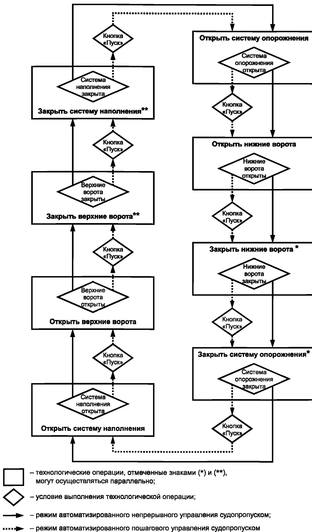
Рисунок 2 — Алгоритм обеспечения последовательности операций по маневрированию исполнительными механизмами для однокамерного шлюза
