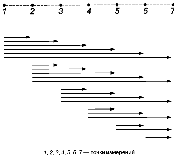
Рисунок 4 — Измеряемые расстояния
