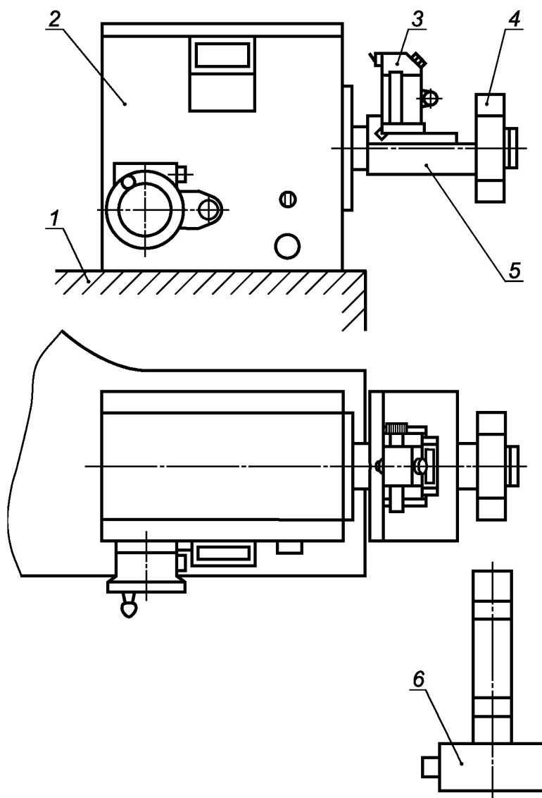
Схема установки для поверки квадрантов
