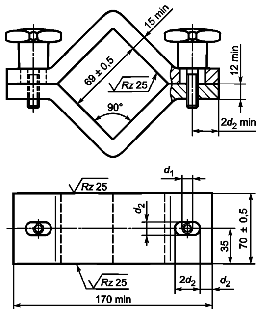
Рисунок 2 — Зажимная форма для установки кубической пробы
