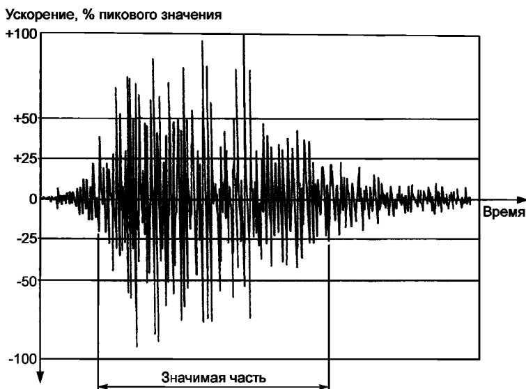
Рисунок 4 — Типичная форма временного сигнала возбуждения
