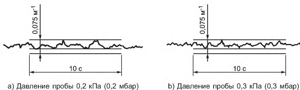
Рисунок 7 — Неустойчивость значений (13.3.2.2)
