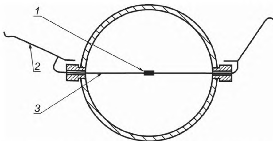
Рисунок 3 — Установка термопары (11.6.1.1)
