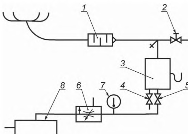
Рисунок 4 — Дымомер с источником света от лампы накаливания (11.6.3)
