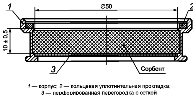
Рисунок 4 — Секция колонки с сорбентом
