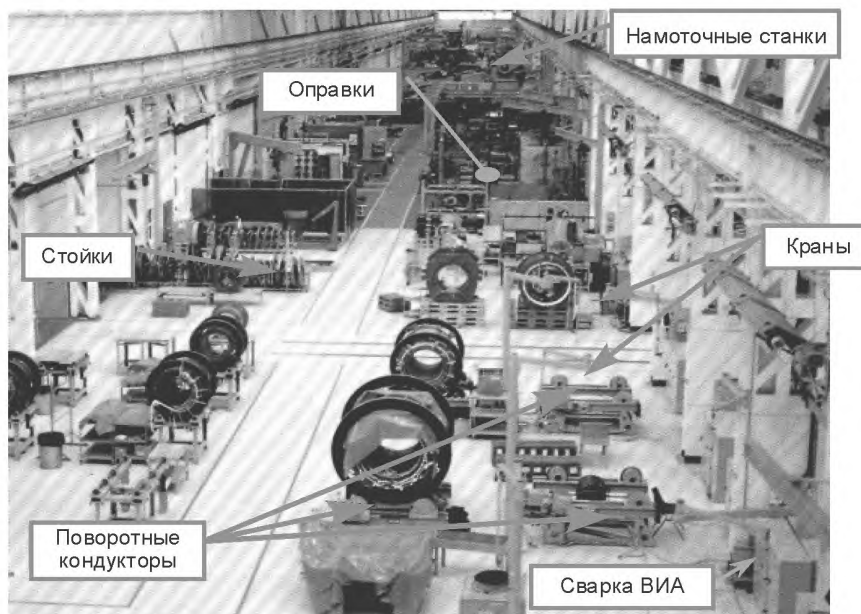
Рисунок В.2 — Пример сборочного цеха
