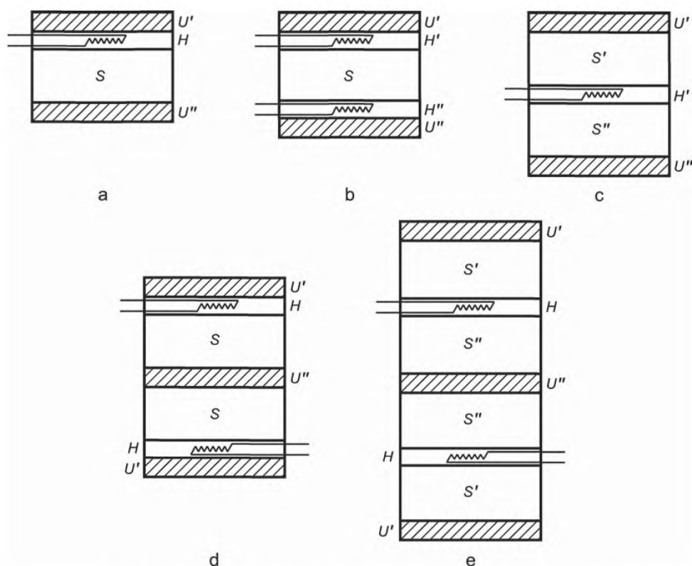
Рисунок 2 — Типовые схемы испытания на приборе, оснащенном тепломером (тепломерами)
