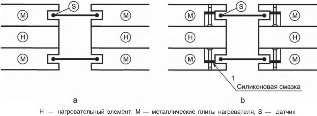
Рисунок Д.3 — Конструктивное решение зазора
