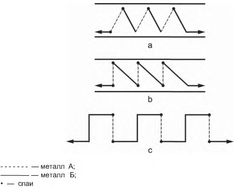
Рисунок D.7 — Примеры расположения спаев термопар термобатареи
