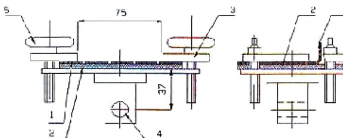
Рисунок А.2 - Струбцина для крепления образцов.
