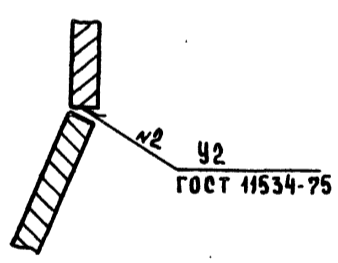
Б-Б М 1:1
