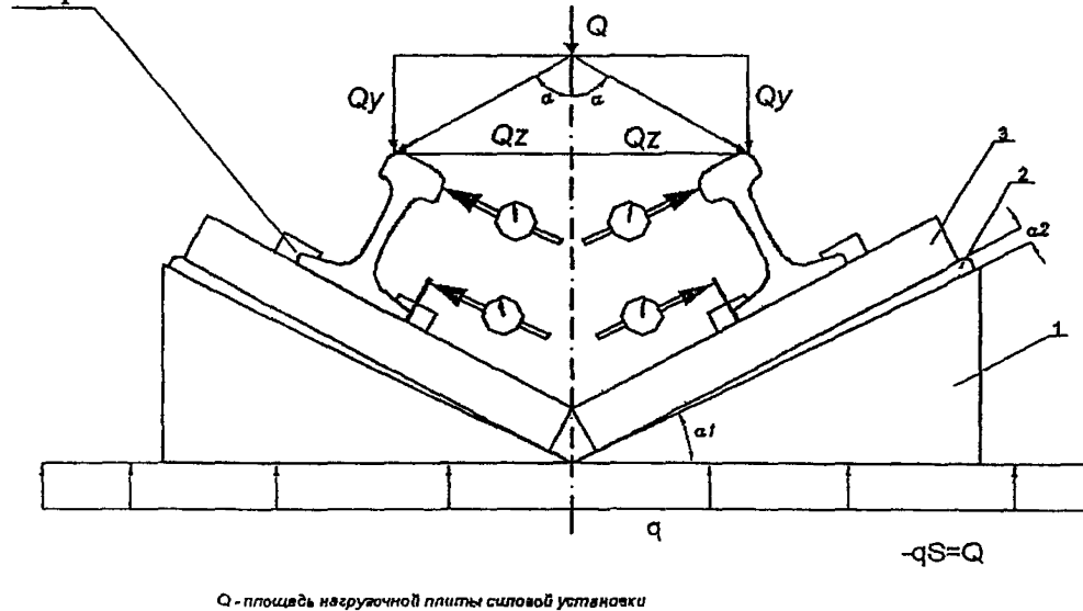
Рисунок А1 – Схема нагружения двух узлов рельсового крепления на испытательной машине
