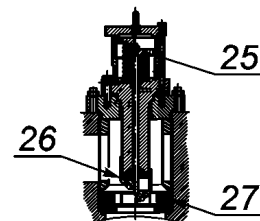
Разгрузочное устройство с затвором
