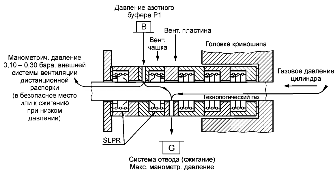
Прижимное уплотнение
