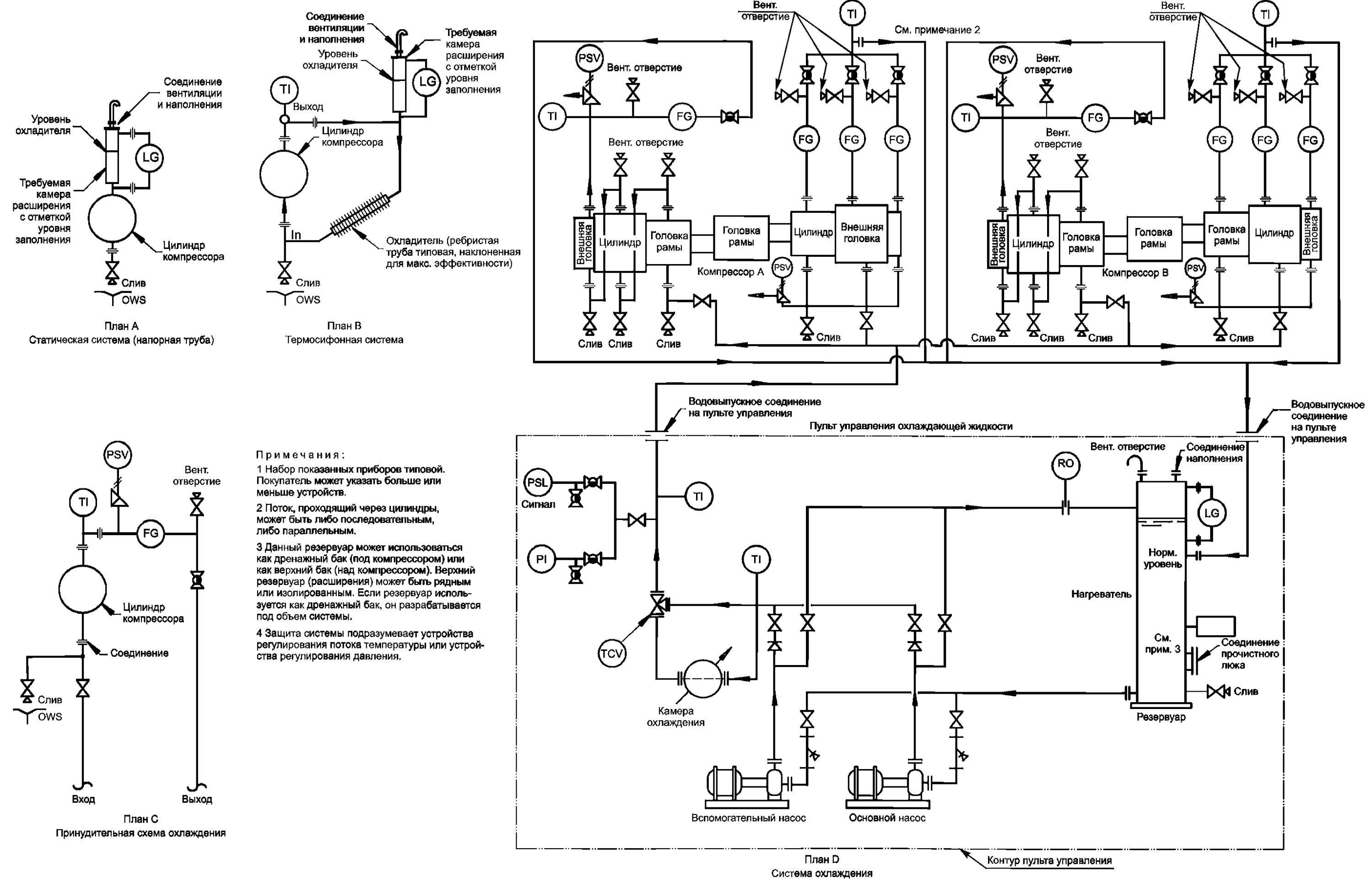
Рисунок G.2 — Схема системы охлаждения цилиндра
