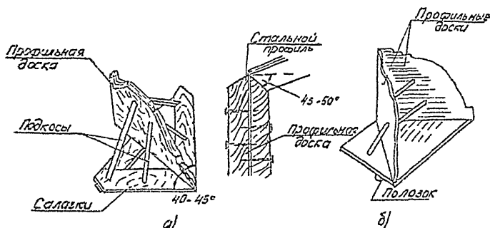
Рис. 7 Угловые шаблоны:
