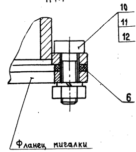
В-В повернуто 1:1
