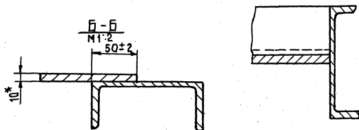
В-В М1:2
