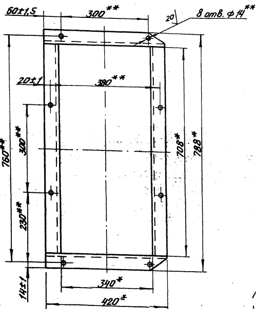
Вид Г Лист 2 детали поз.7,8,13,16,21 условно не показаны.
