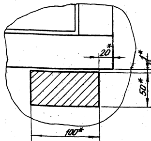
Д-Д повернуто Лист 2 М1:2
