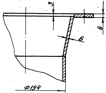
Г-Г лист 1 М1:2
