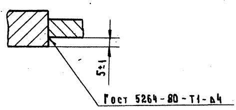
6-6 ПОВЕРХНО
