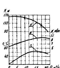
Характеристика насоса 33ЦДБ8-16-140
