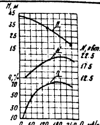
Характеристика насоса 34.5 12-210-25
