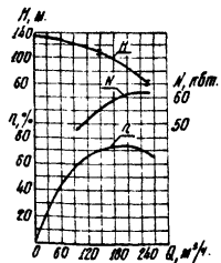
Характеристика насоса 234.5 12-210-65
