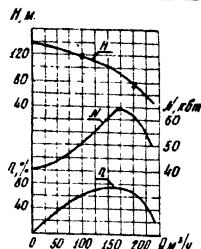
Характеристика насоса 34.5 12-160-100
