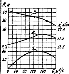
Характеристика насоса 34.5 10-160-35Г
