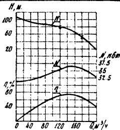
Характеристика насоса 34.5 10-160-65
