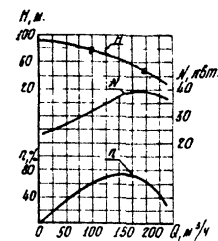
Характеристика насосов 34.5 12-160-65 и 234.5 12-160-65
