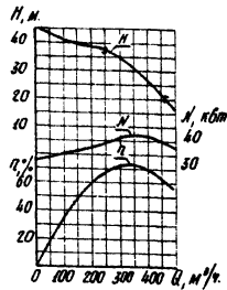
Характеристика насоса 34.5 12-315-30
