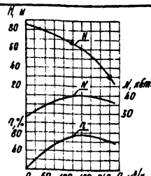
Характеристика насоса 34.5 12-210-55
