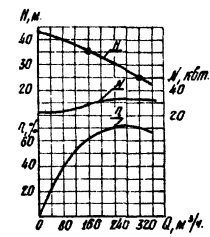
Характеристика насоса 234.5 12-255-30Г
